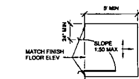
3 TYP STOOP 1/4" = 1'-0"
