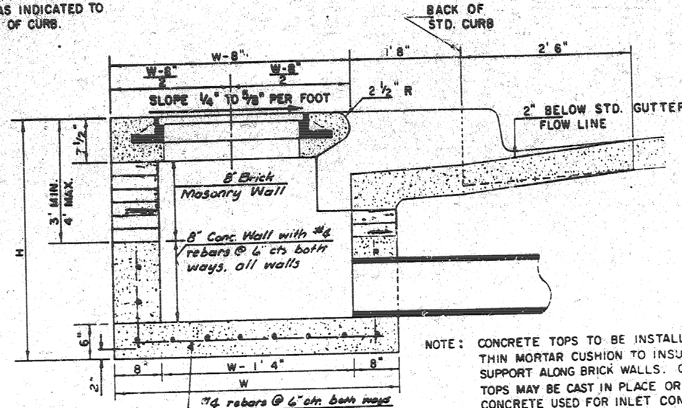
SECTION A-A
