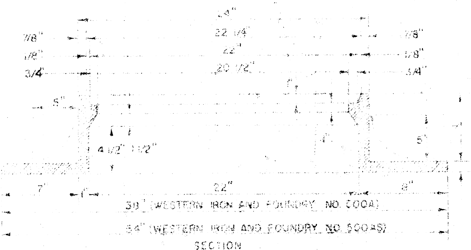
MANHOLE RING
