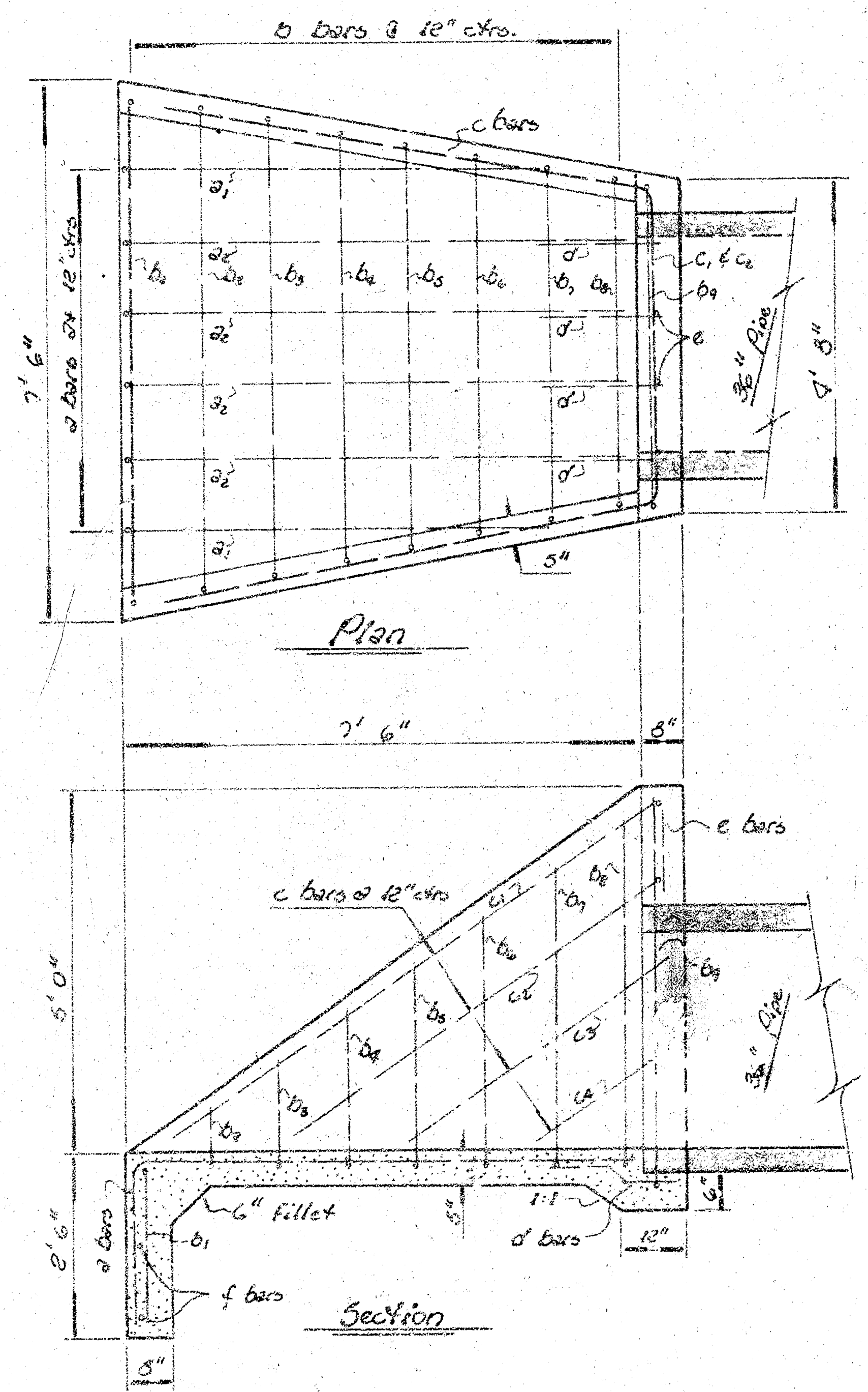
Headwall Scale: 1/8" = 1'
