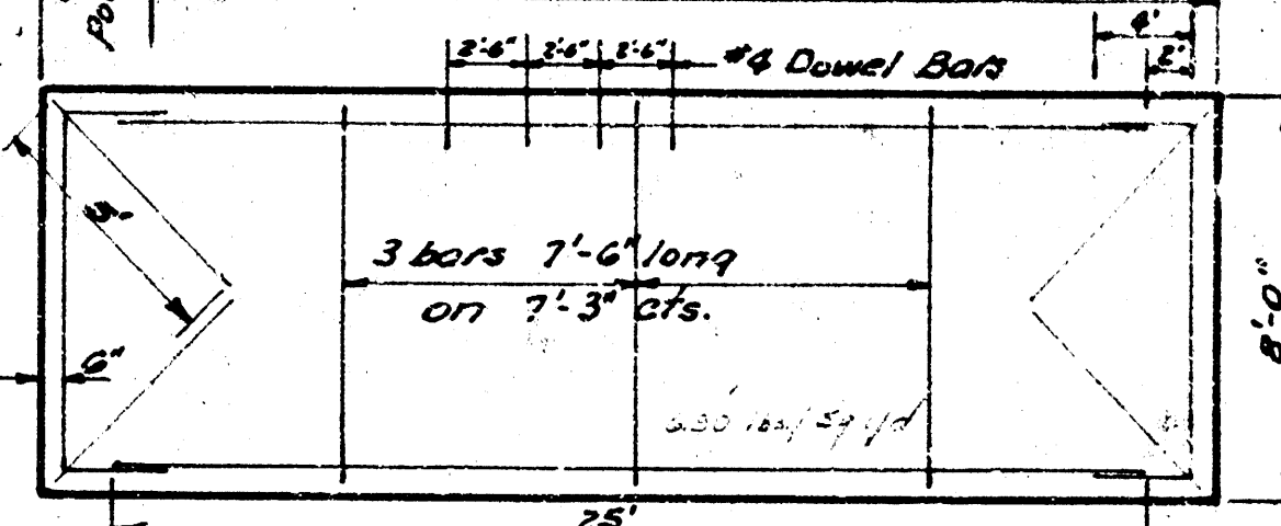
STEEL PATTERN No Scale:
