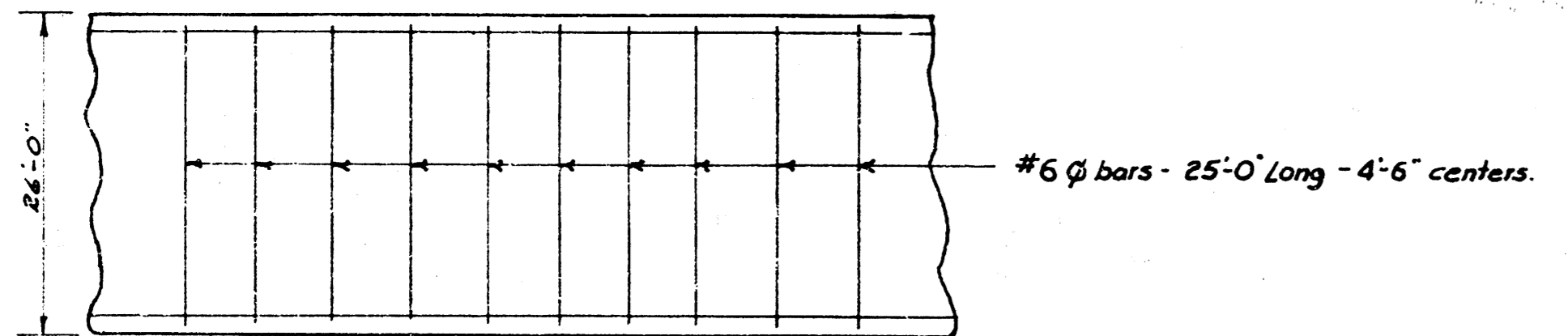
TYPICAL STEEL PATTERN Sta. 0+00 to Sta. 5+05.19 No Scale.
