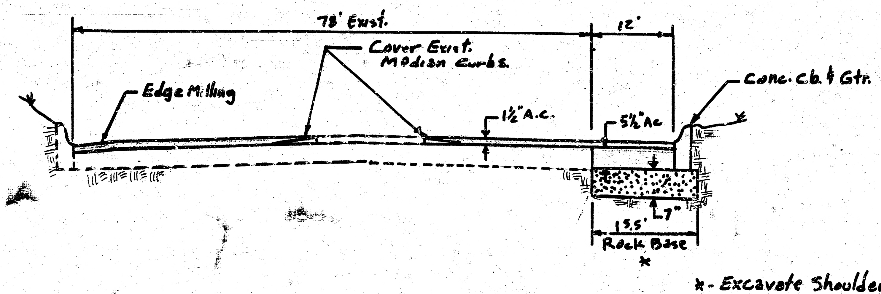
SECTION A-A
