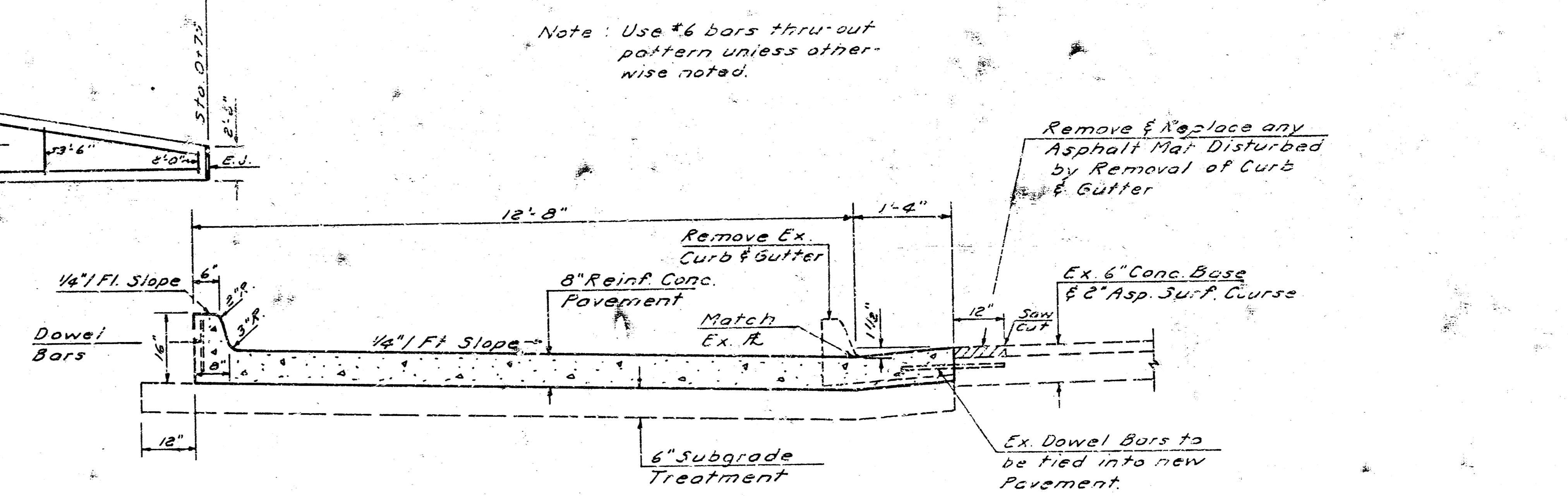
SECTION A-A
