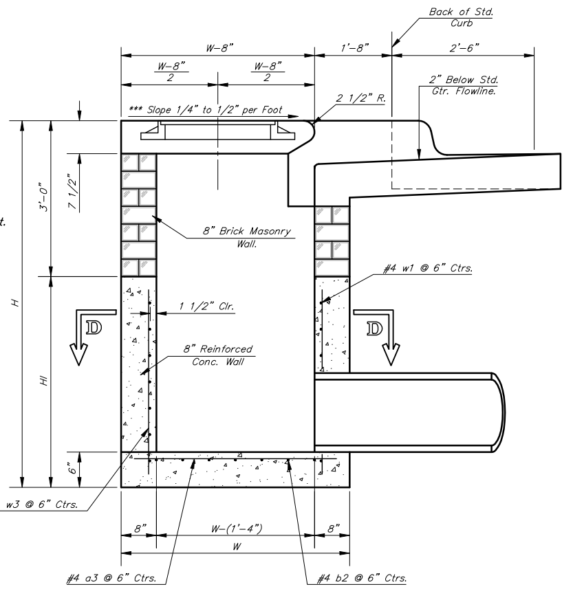
SECTION A-A
