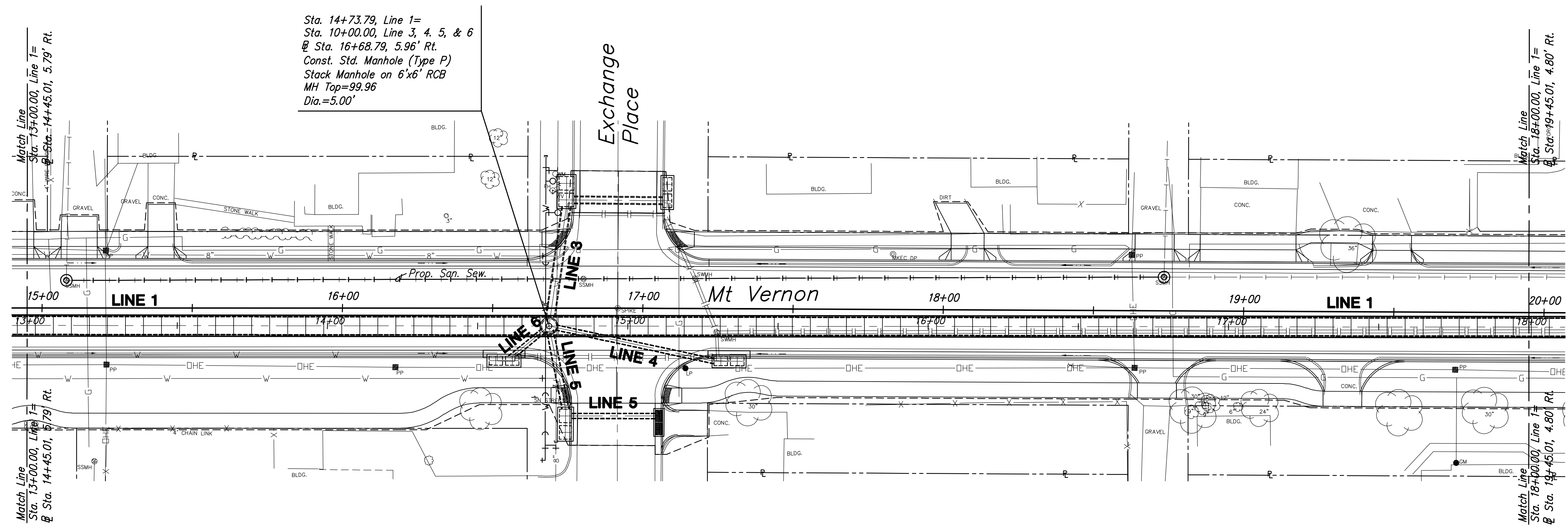
PLAN-LINE 1 SCALE: 1"=20'
