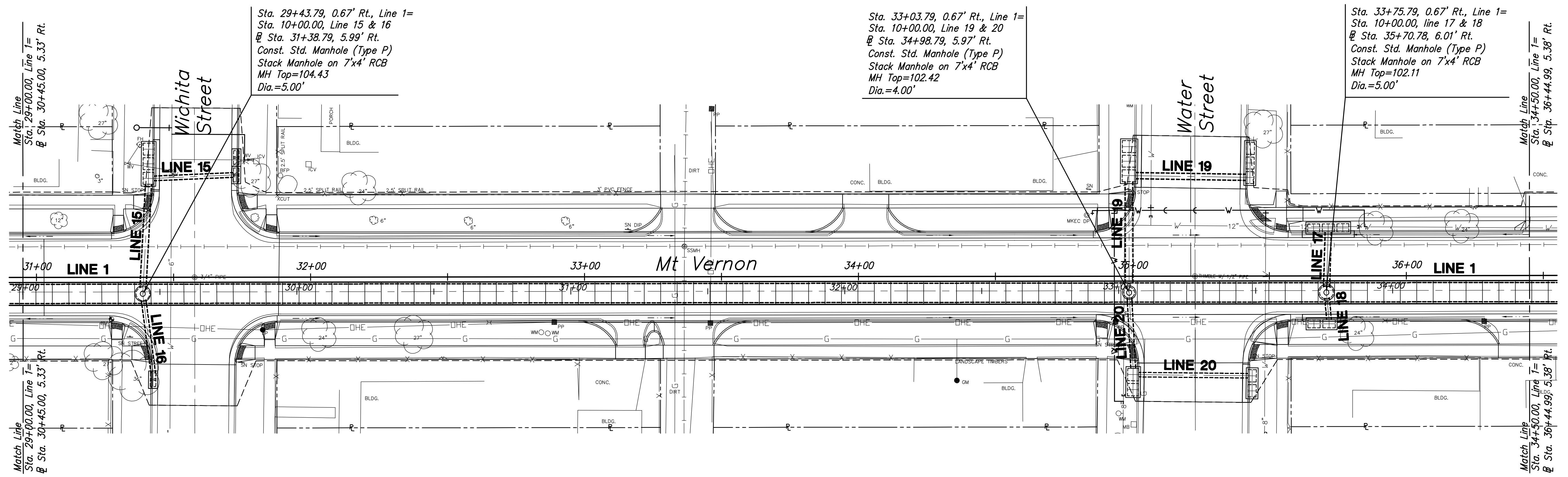
PLAN-LINE 1 SCALE: 1"=20'
