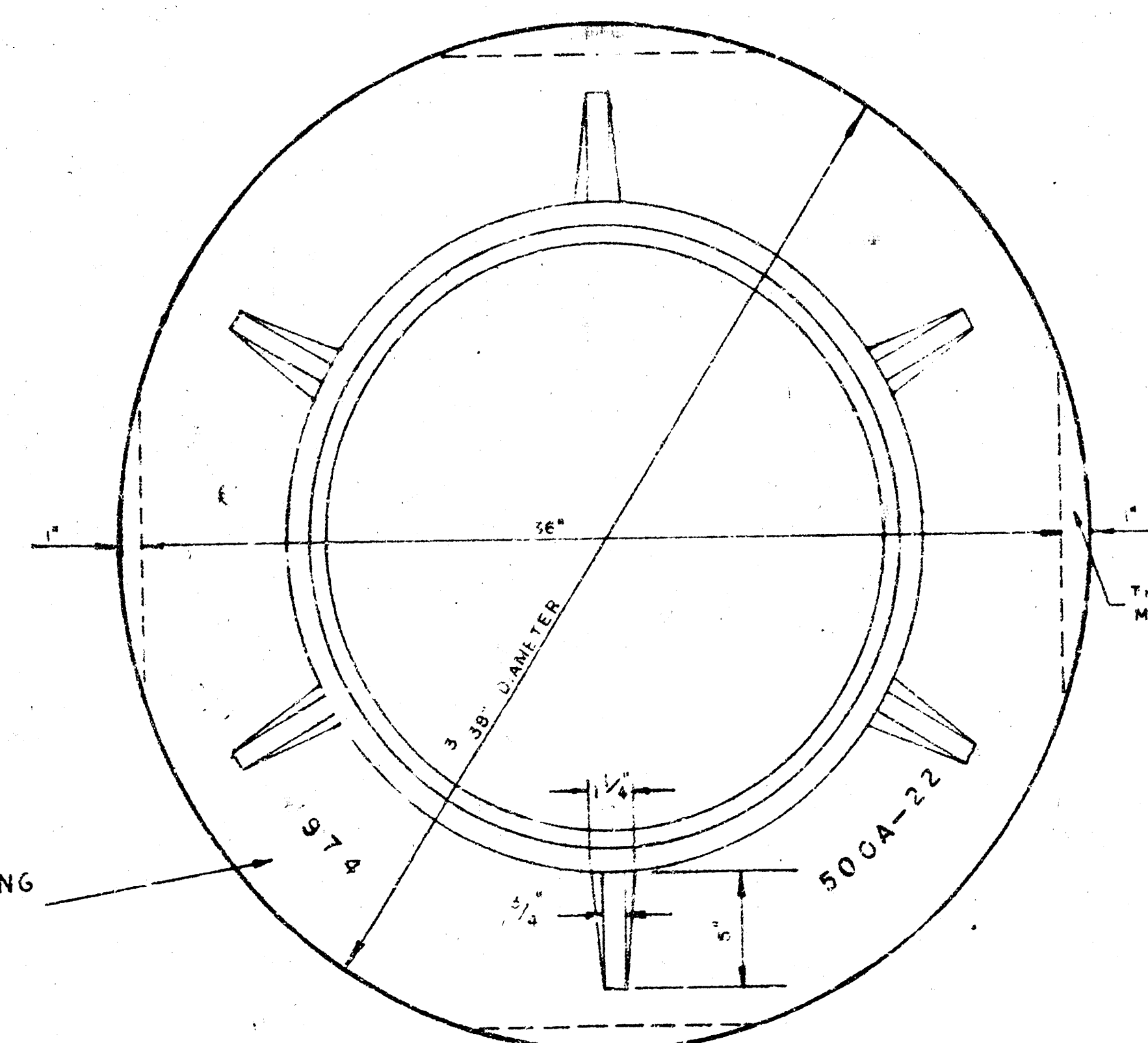
MANHOLE RING
