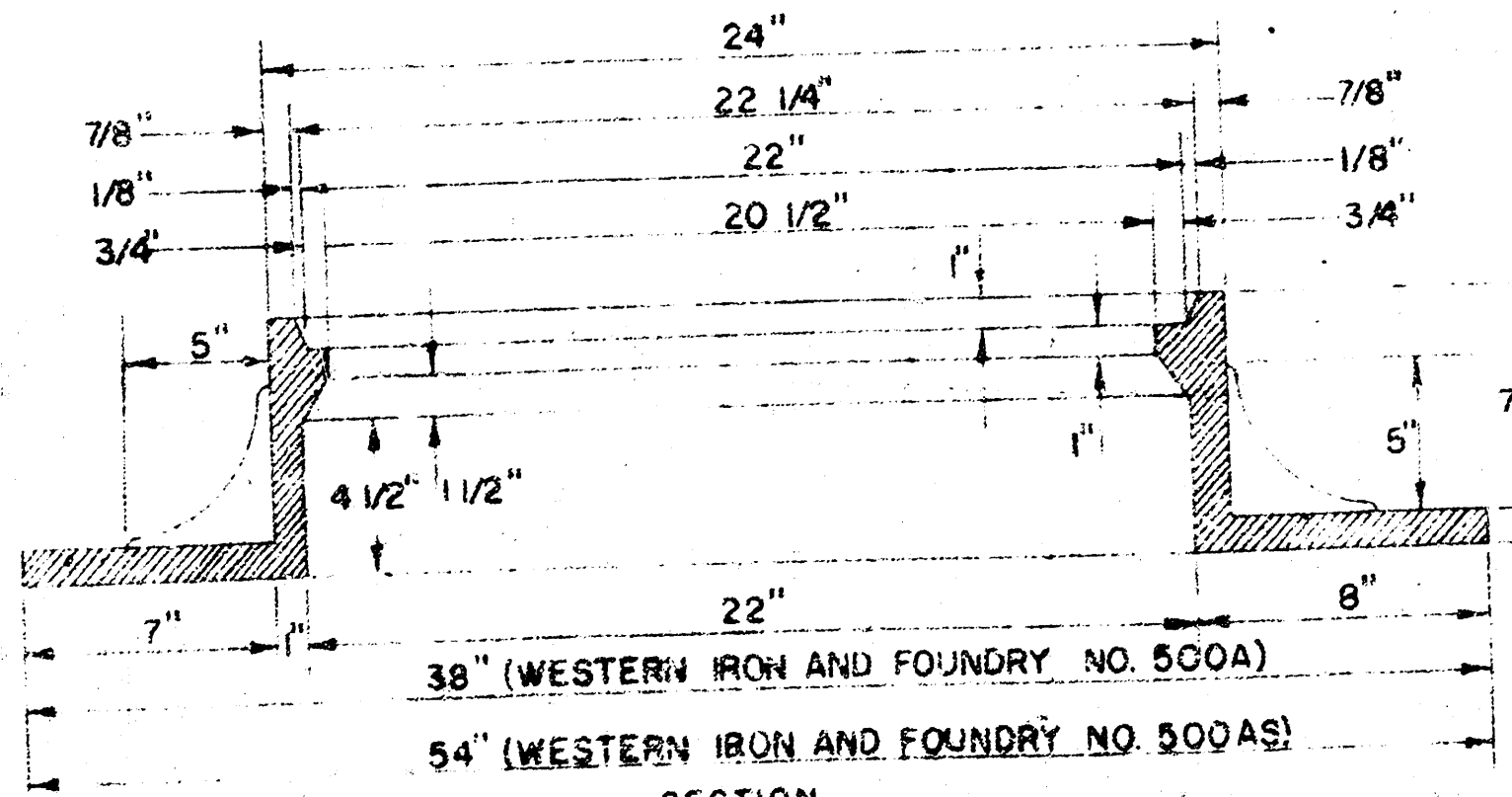
MANHOLE RING
