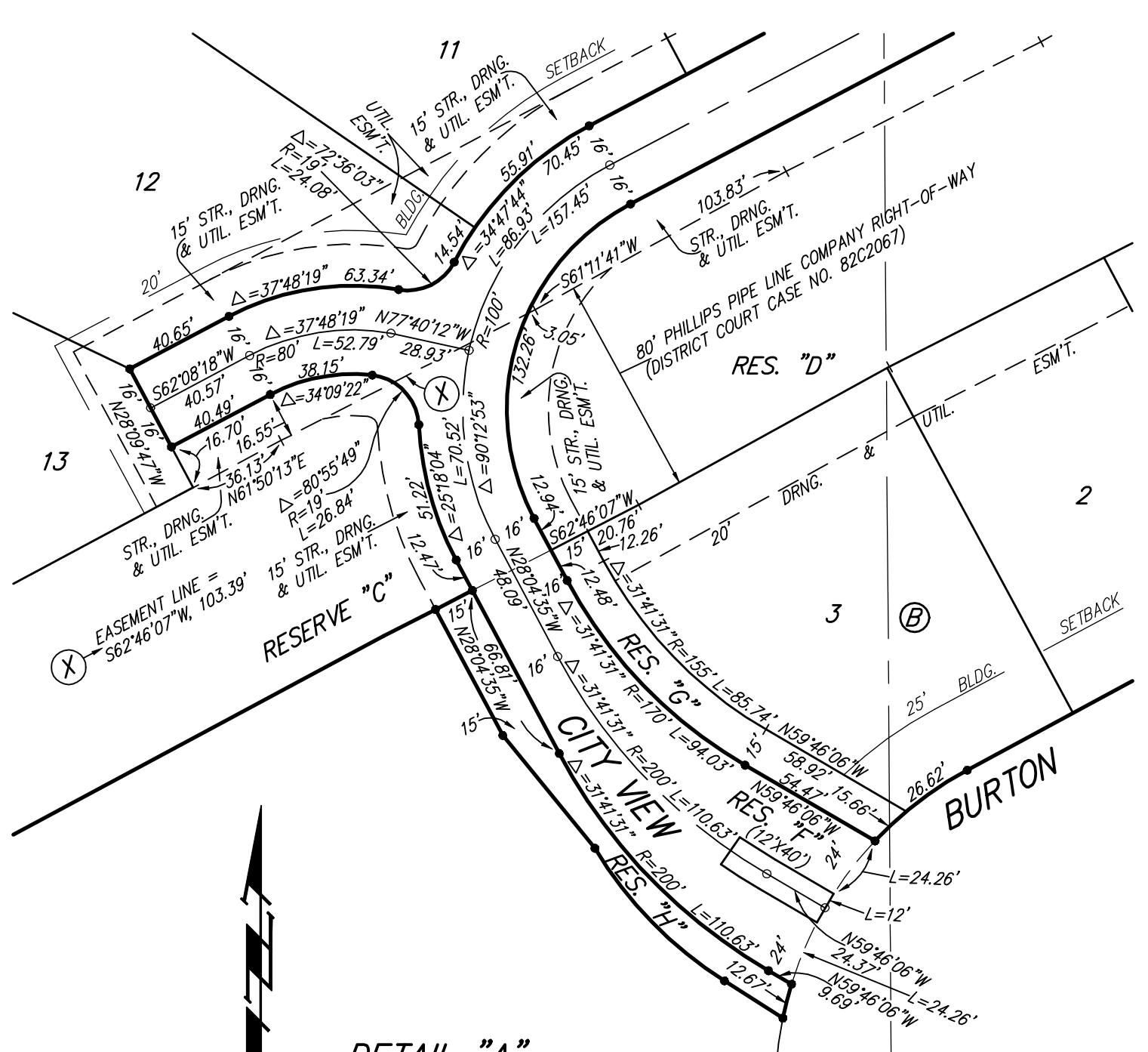
DETAIL "A" (NO SCALE)
