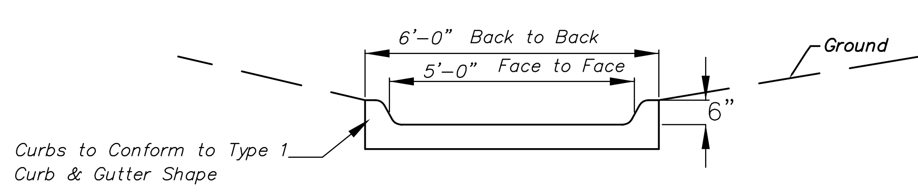
SECTION A-A INLET FLUME DETAIL N.T.S.
