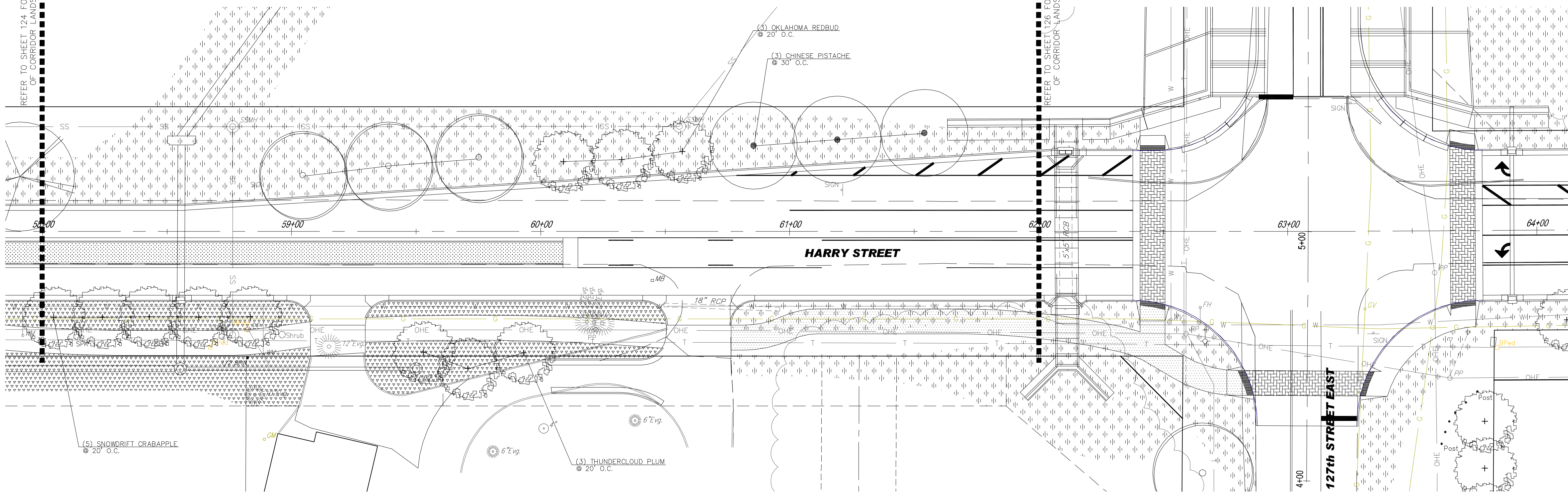
LANDSCAPE PLAN Sta 58+00 to Sta 62+00
