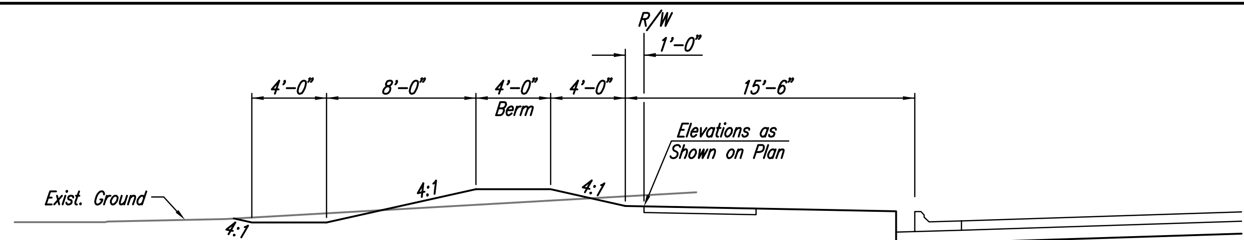
SECTION A-A Sta. 11+90± to Sta. 13+00± See Cross Sections
