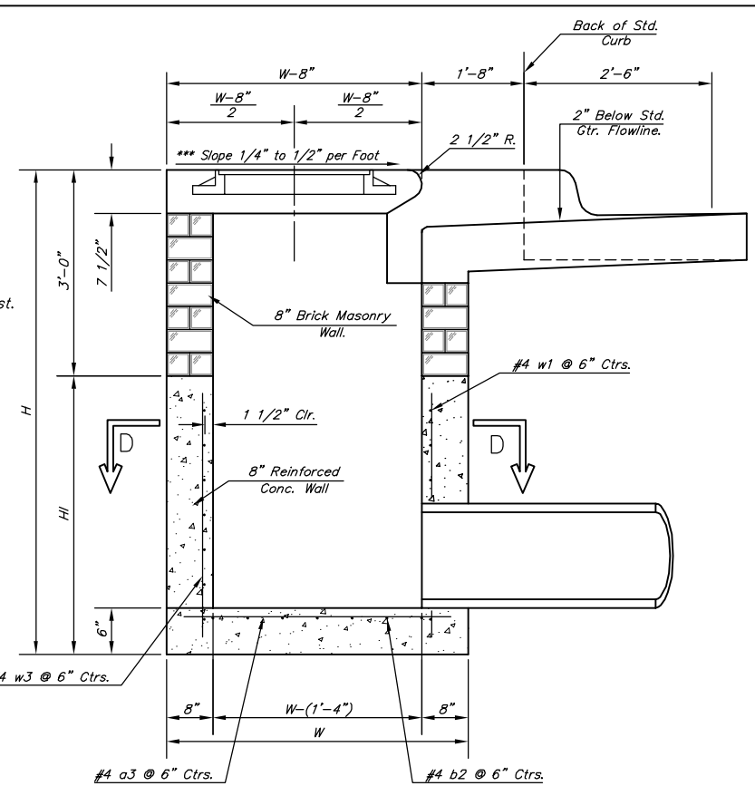
SECTION A-A
