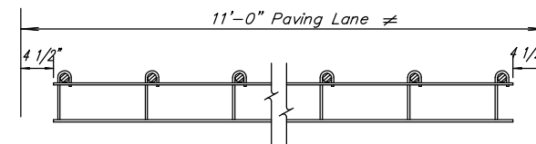
SEC. A-A
