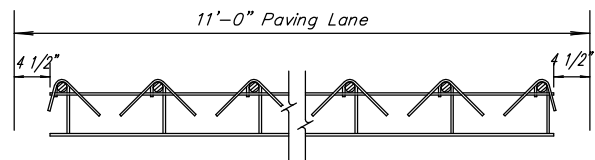
SEC. A-A
