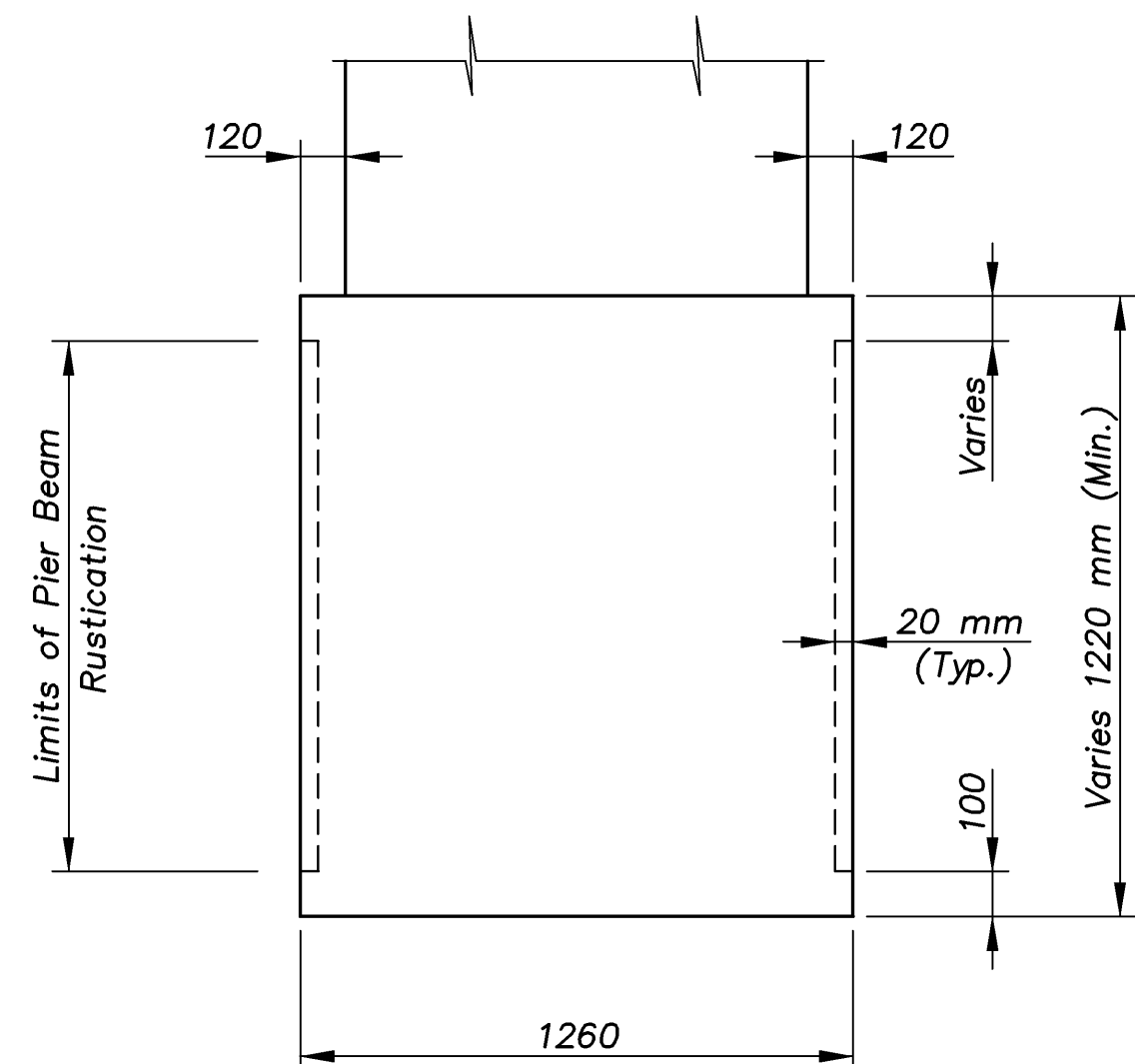
SECTION A-A
