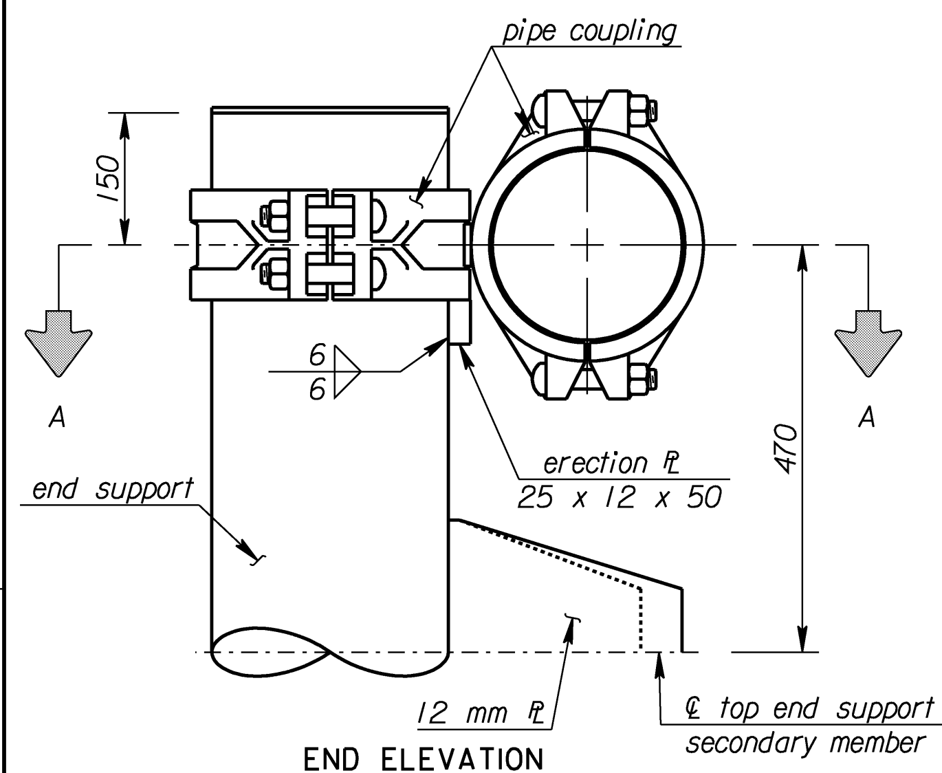
END ELEVATION
