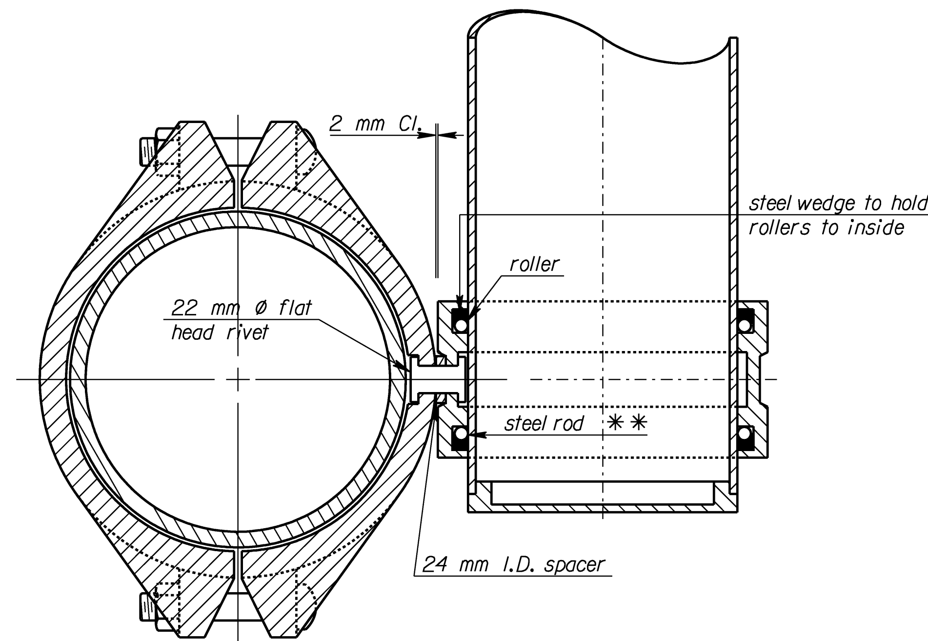
SECTION A-A
