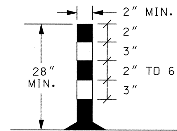
TUBULAR MARKERS
