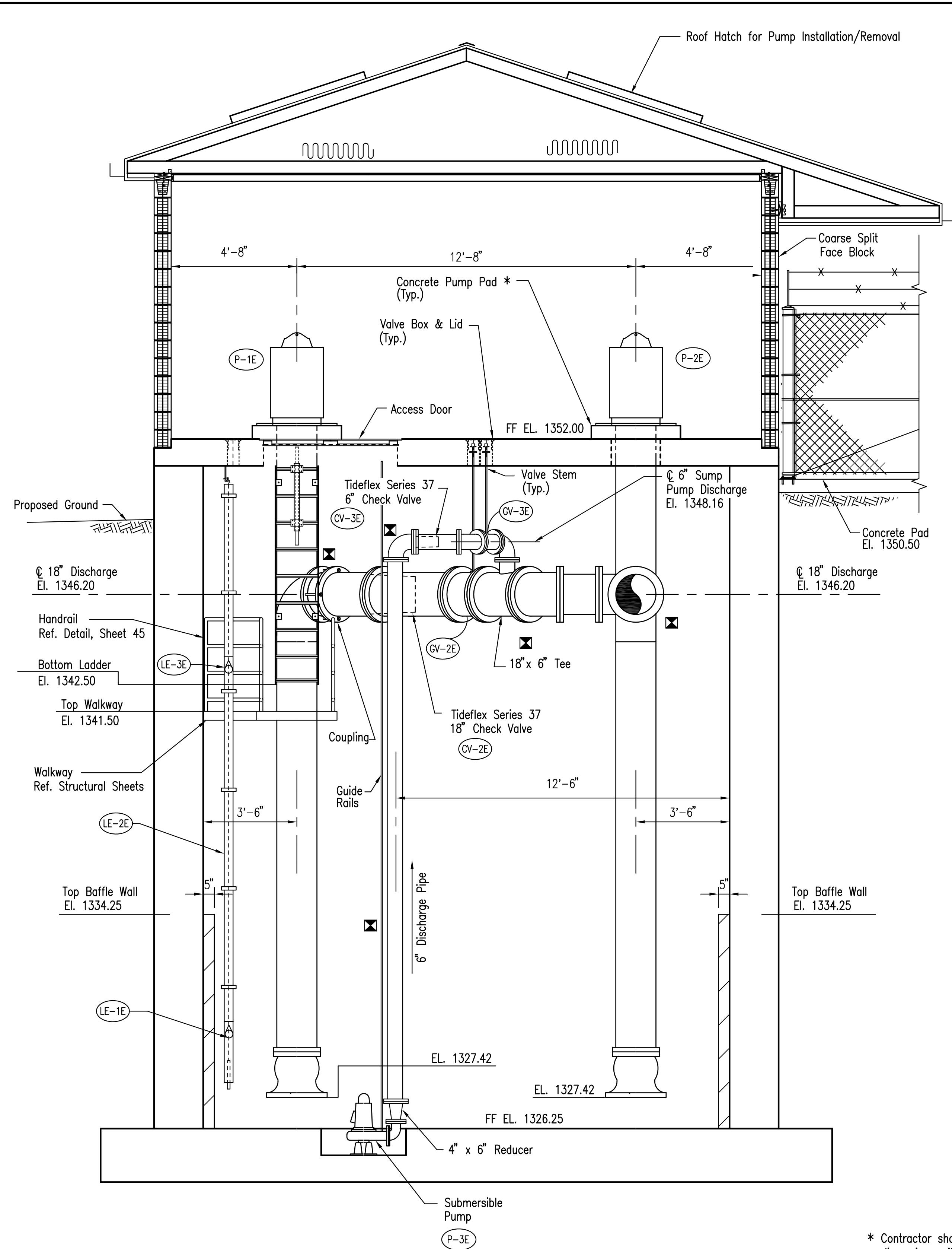
1 SECTION 35 SCALE: 3/8" = 1'-0" 0 1 2 3 4
