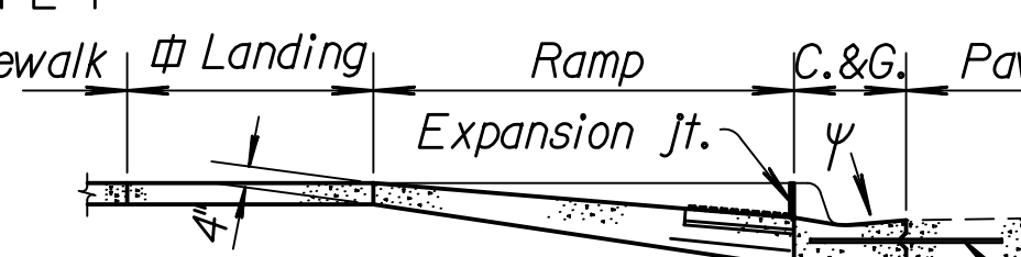
SECTION D-D
