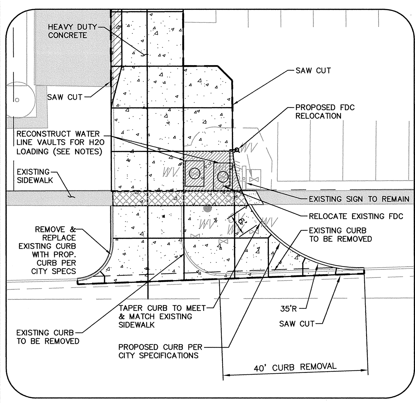
ALLEY DRIVE DETAIL N.T.S.
