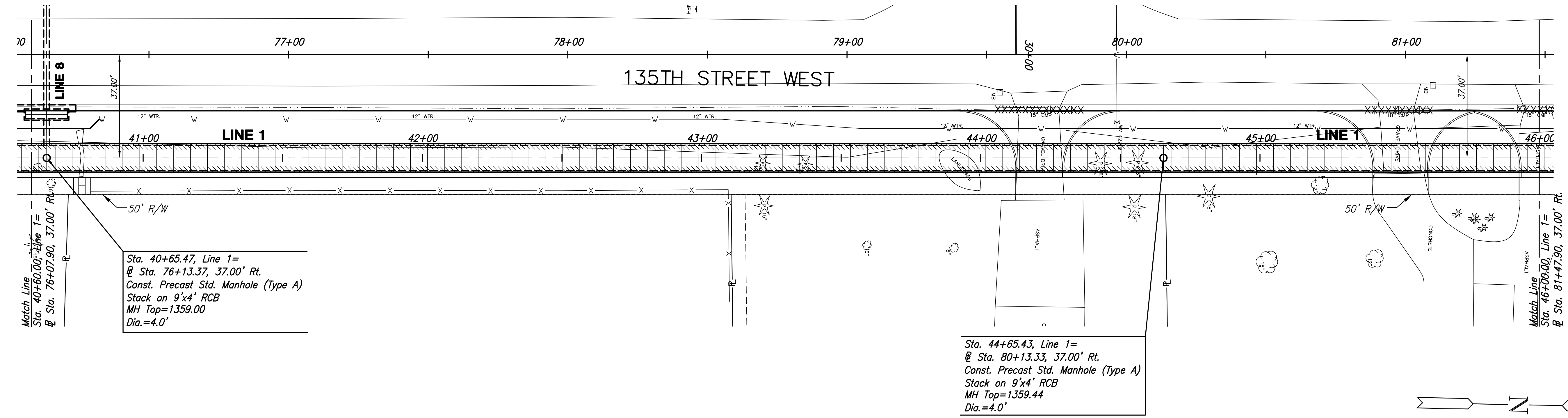
PLAN LINE 1 SCALE: HORIZ. 1"=20' SCALE: VERT. 1"=5'
