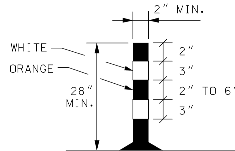
TUBULAR MARKER
