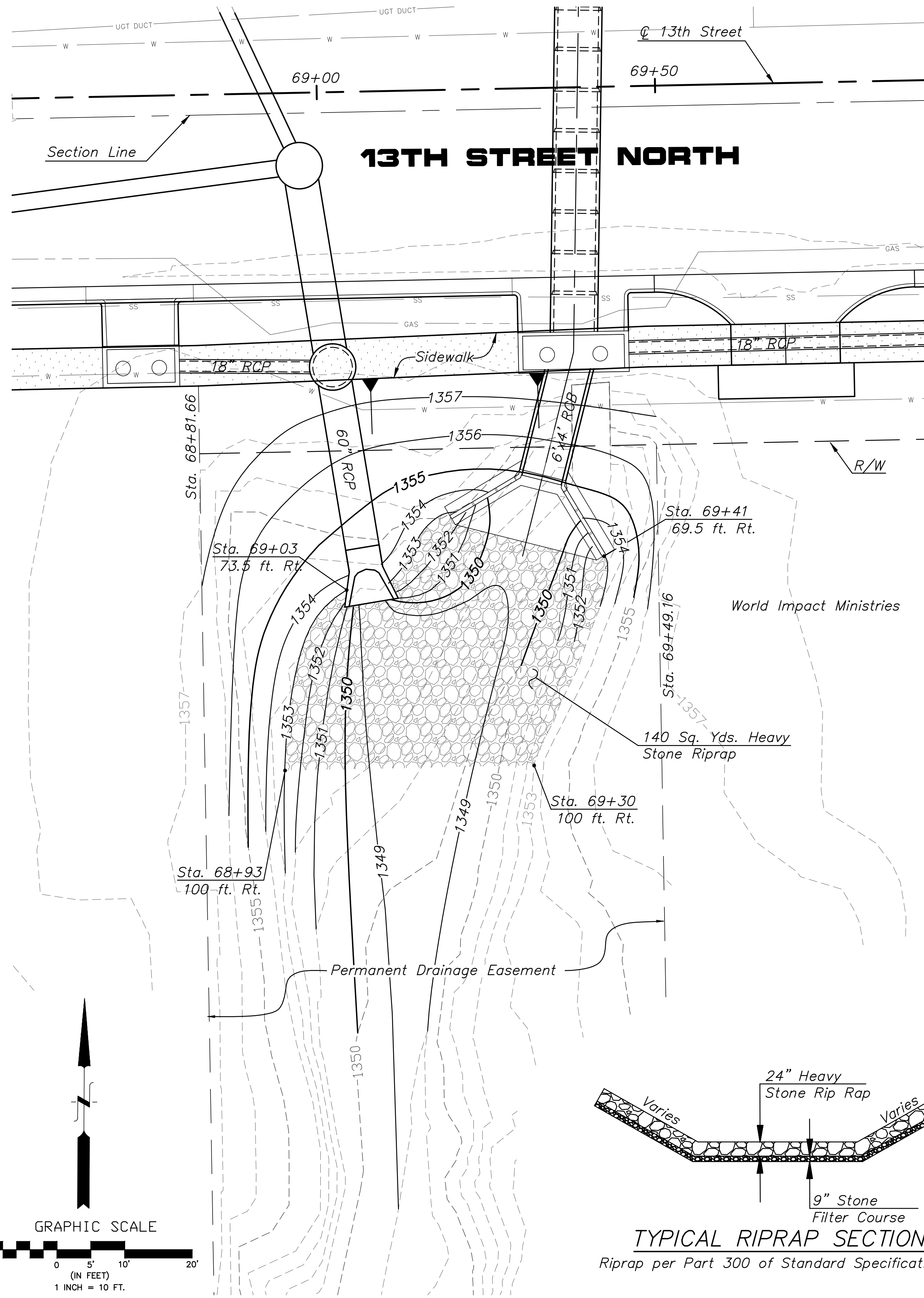
CONTOUR MAP 6'X4' RCB STA. 69+38
