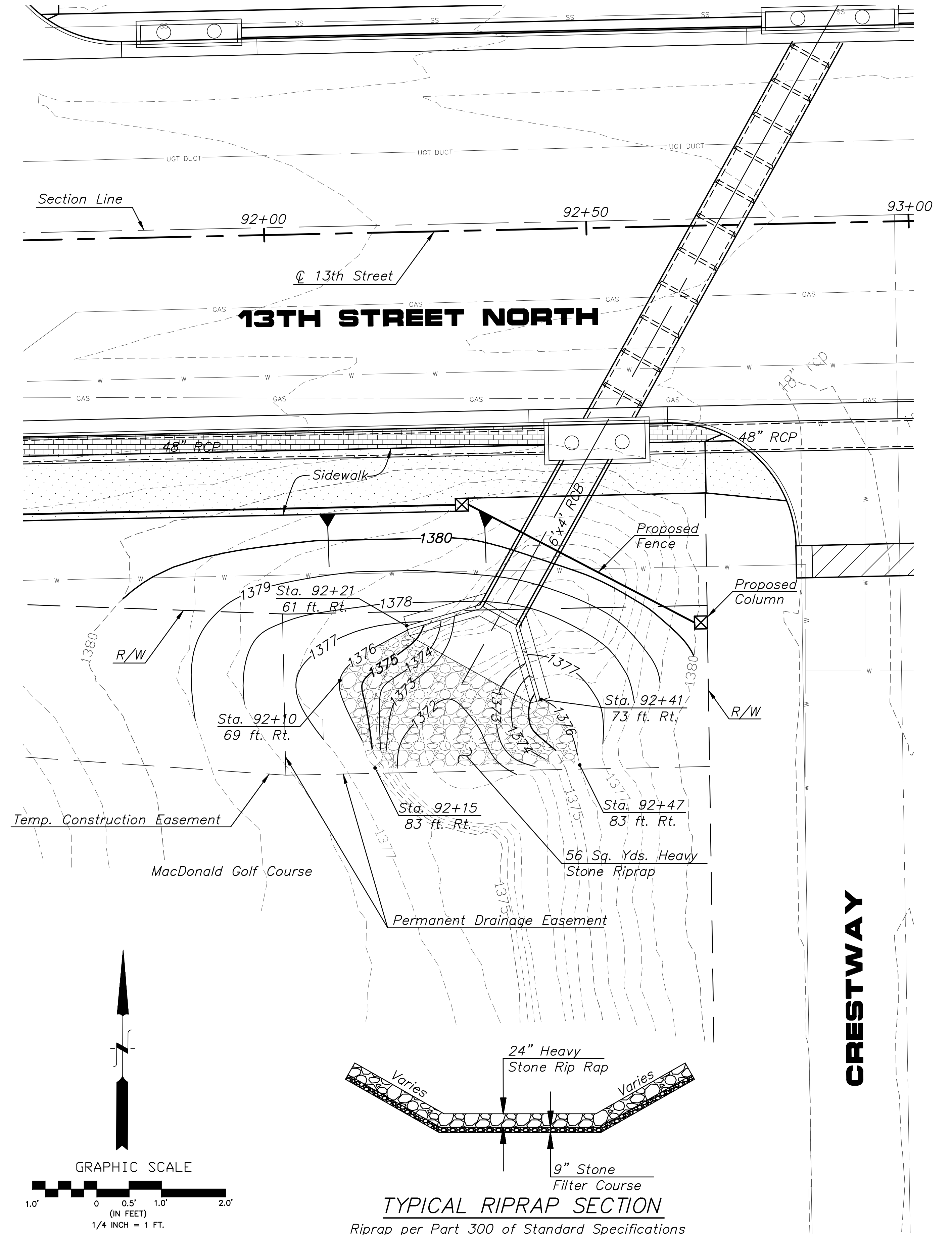
CONTOUR MAP 6'X4' RCB STA. 92+50
