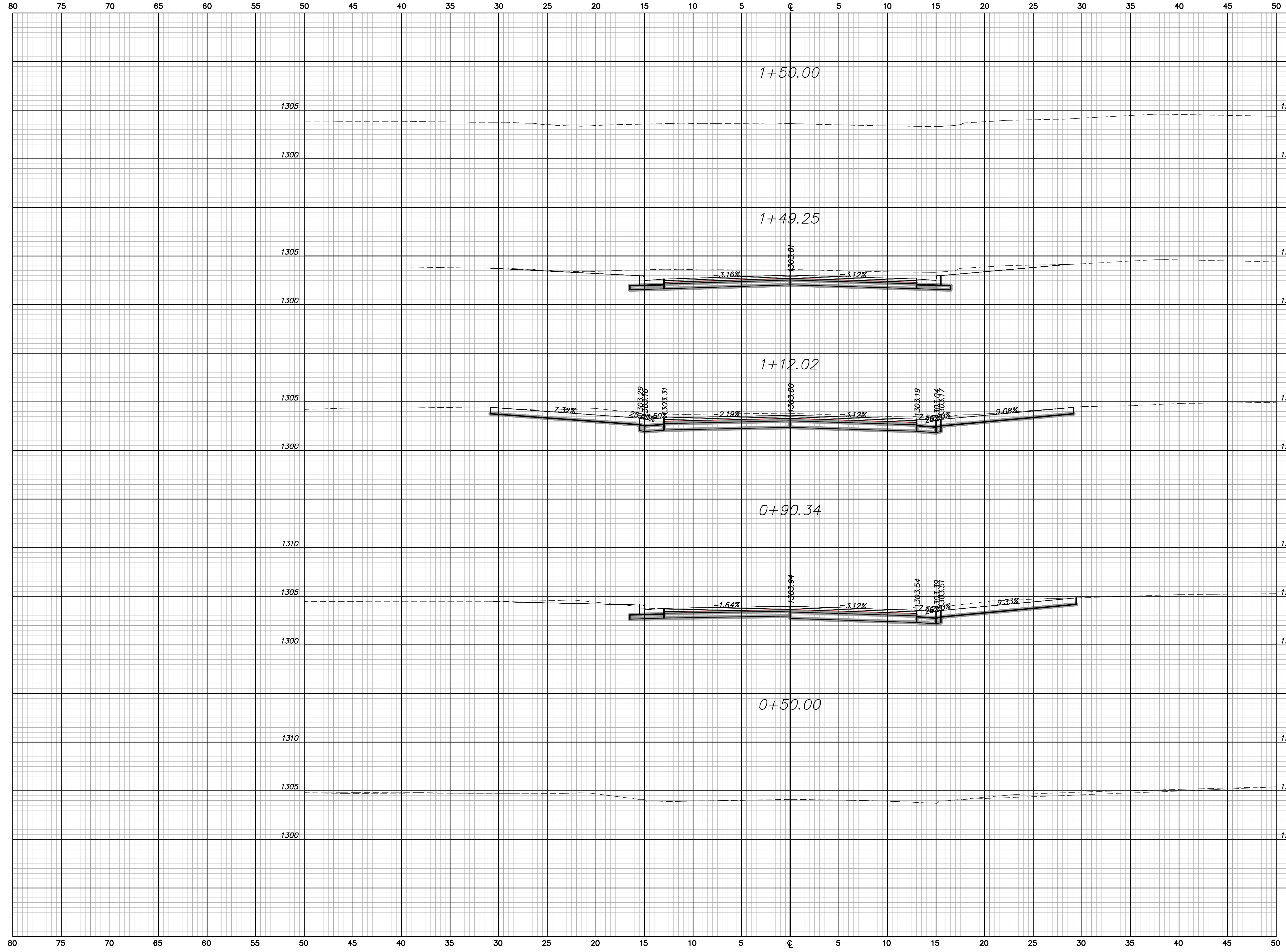
PIATT CROSS SECTIONS Sta. 0+50.00 to Sta. 1+50.00
