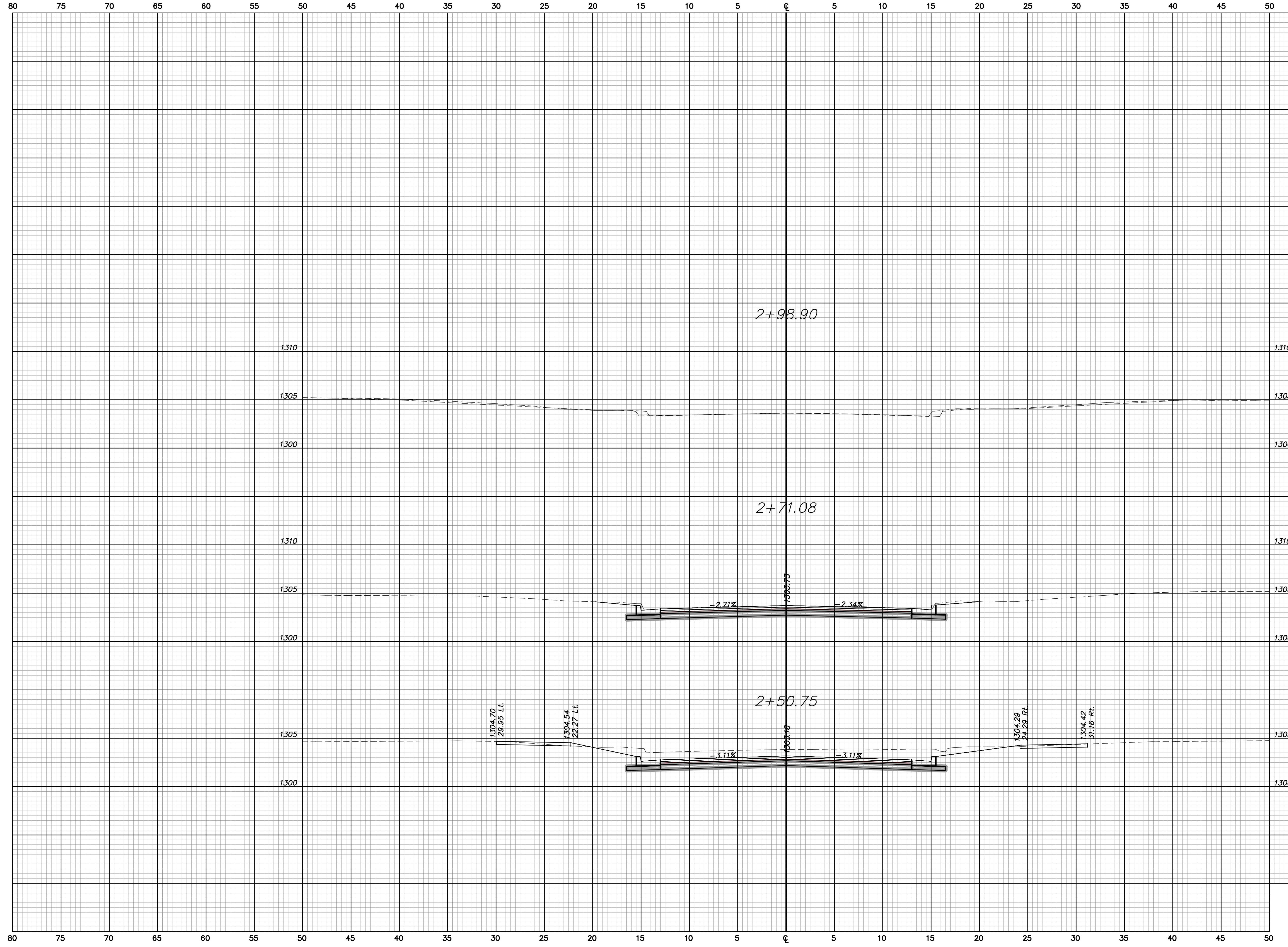
PIATT CROSS SECTIONS Sta. 2+50.75 to Sta. 3+00.00
