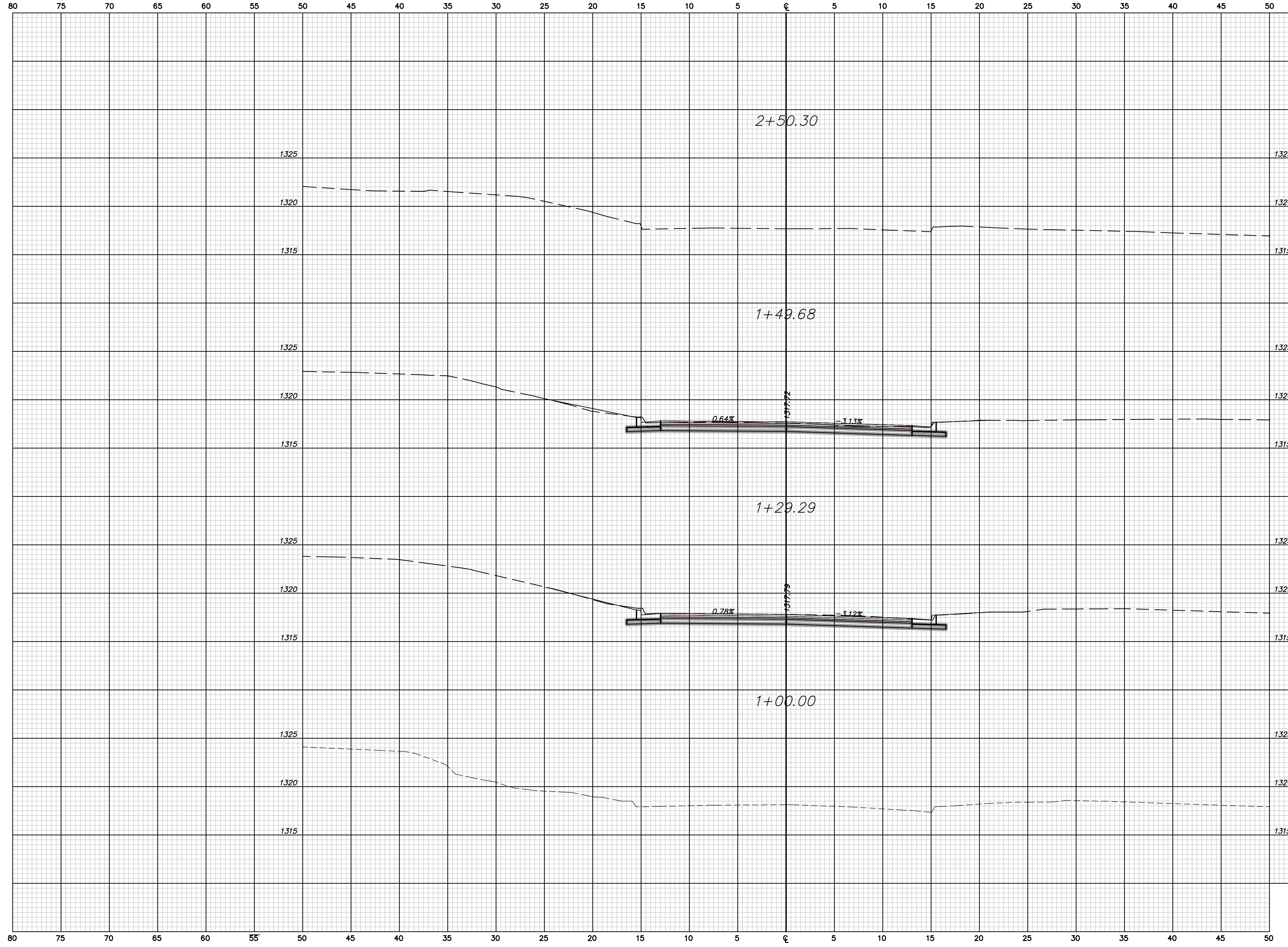
ESTELLE CROSS SECTIONS Sta. 1+00.00 to Sta. 2+50.30
