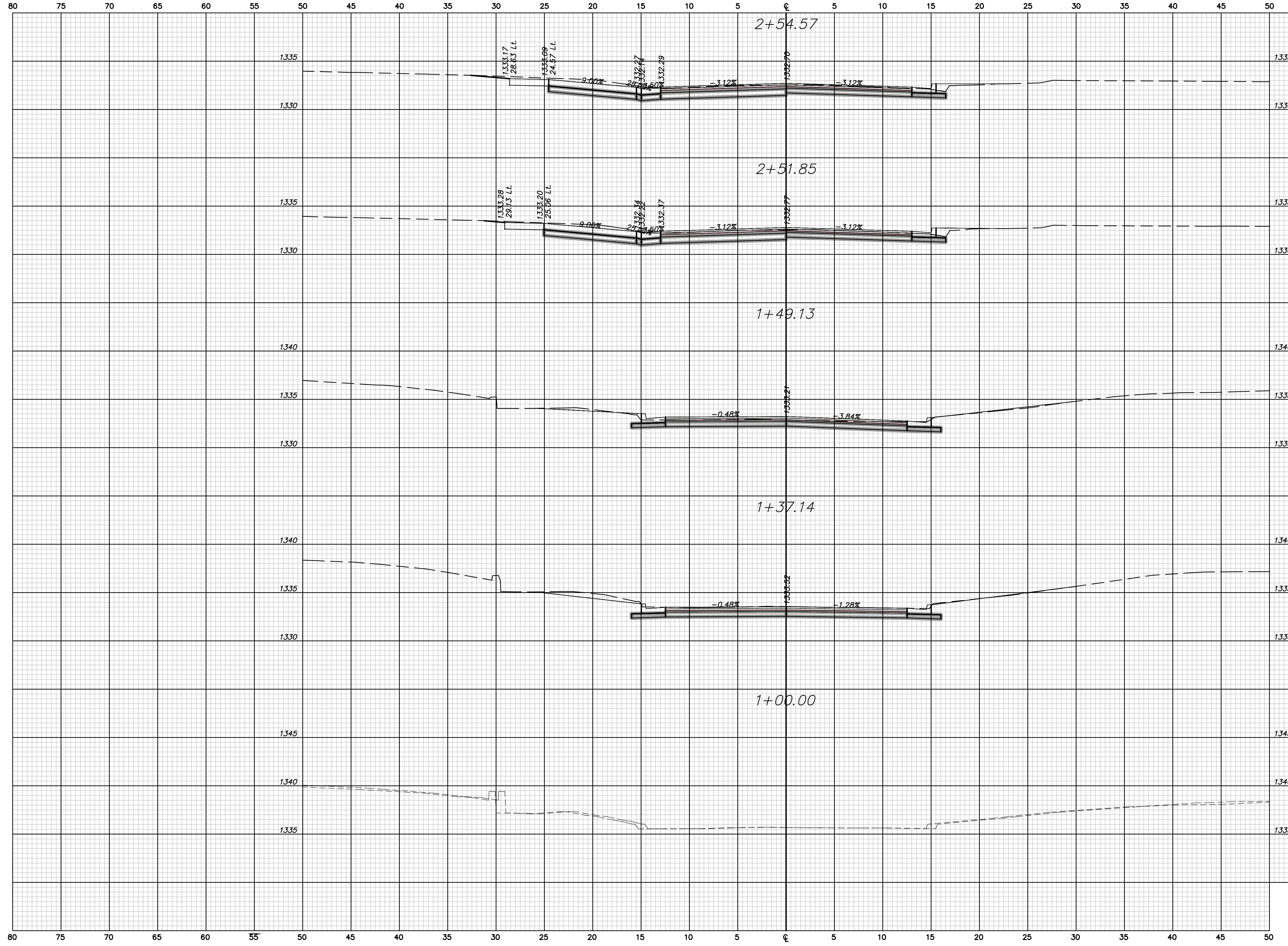
ERIE CROSS SECTIONS Sta. 1+00.00 to Sta. 2+54.57
