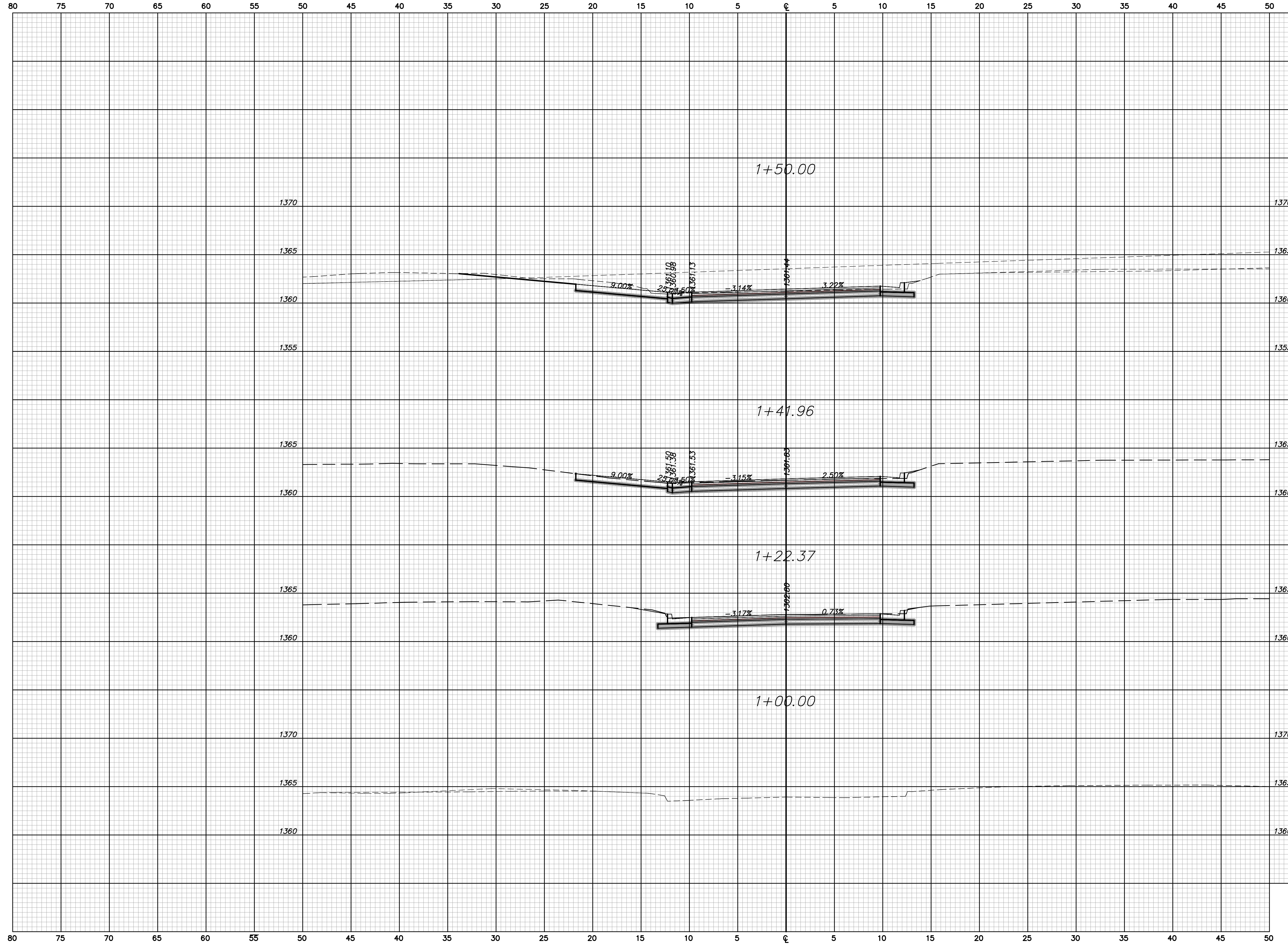
YALE (N. OF 13th ST.) CROSS SECTIONS Sta. 1+00.00 to Sta. 1+50.00
