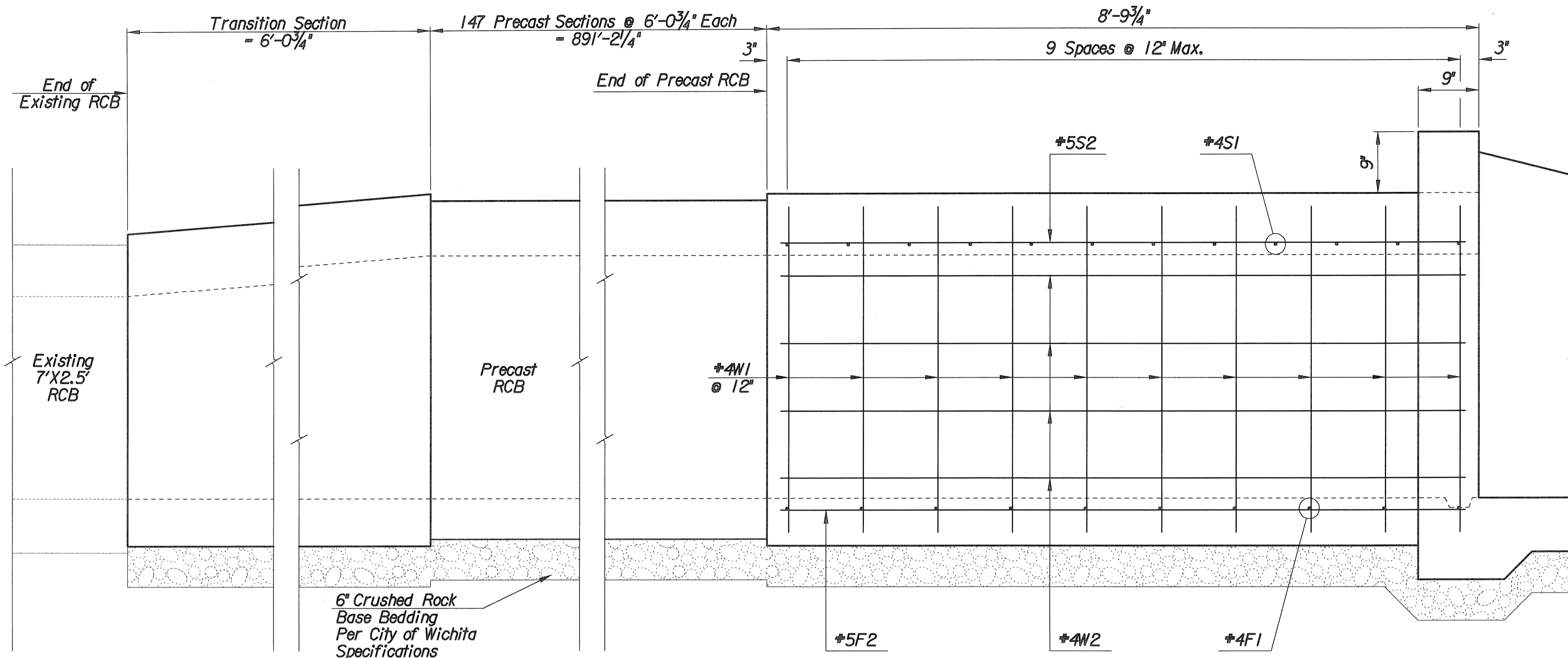
ELEVATION
