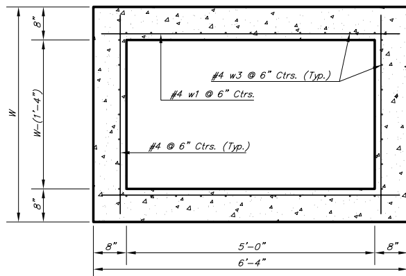
SECTION D-D
