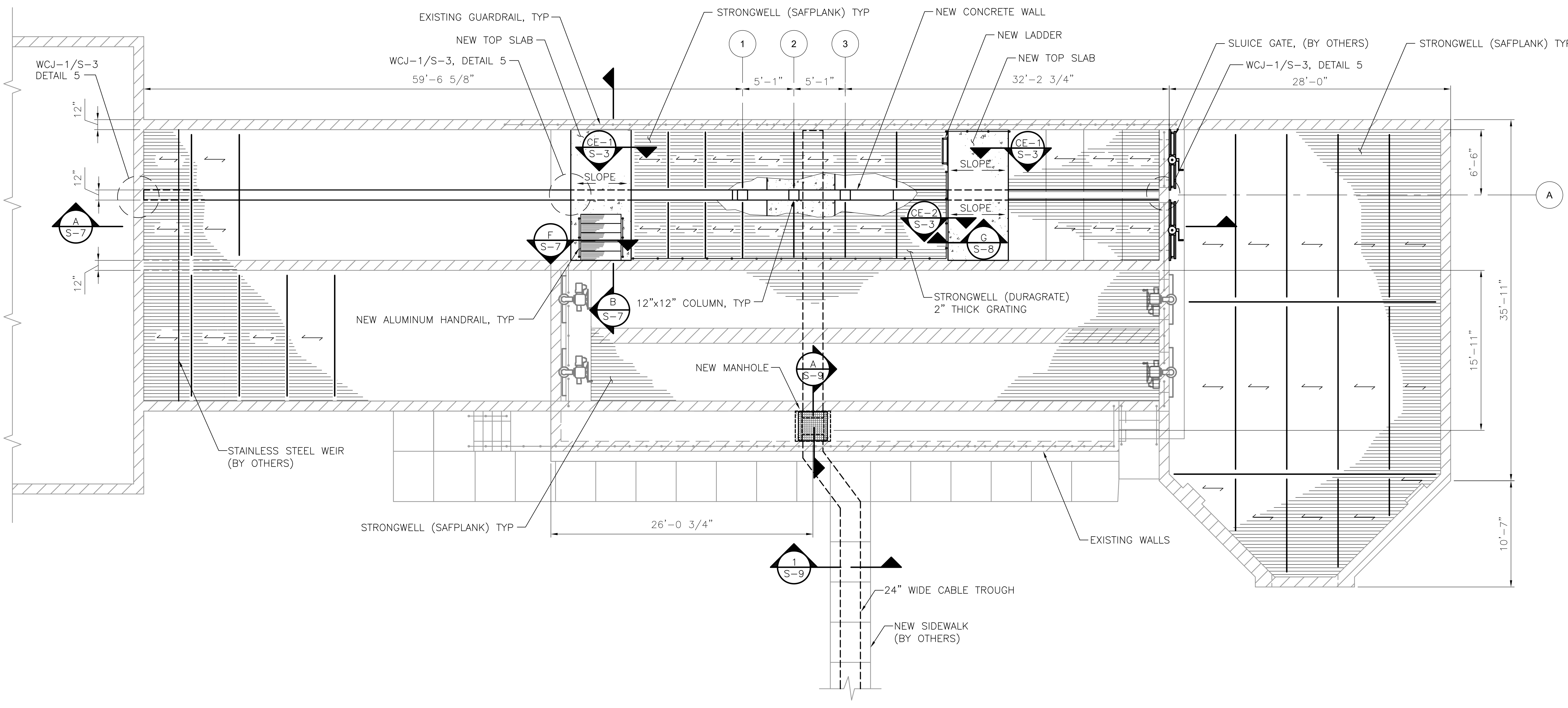
TOP - EL 1267.00 PLAN 3/16" = 1'-0"
