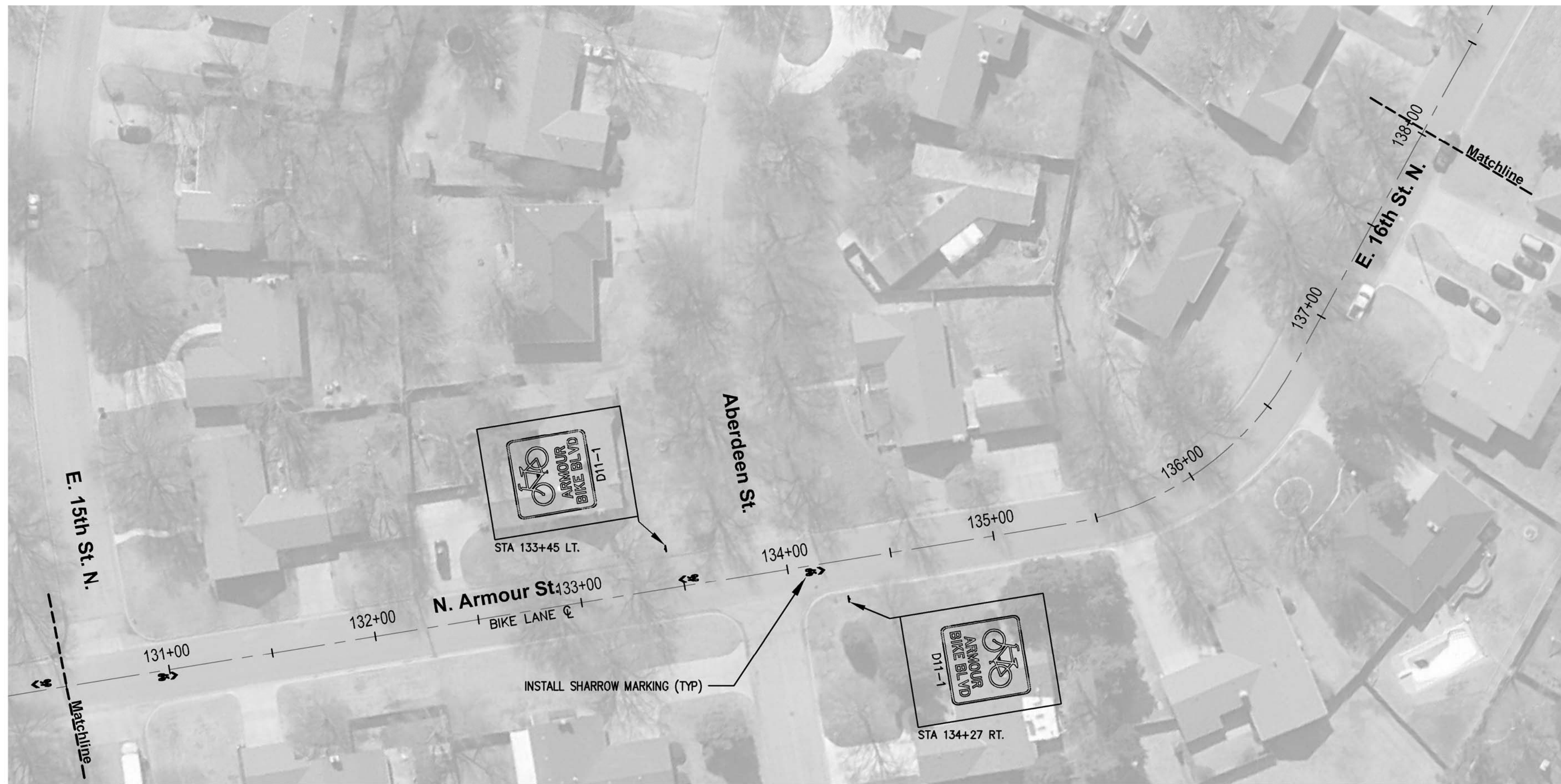
STA 130+50 TO STA 138+00
