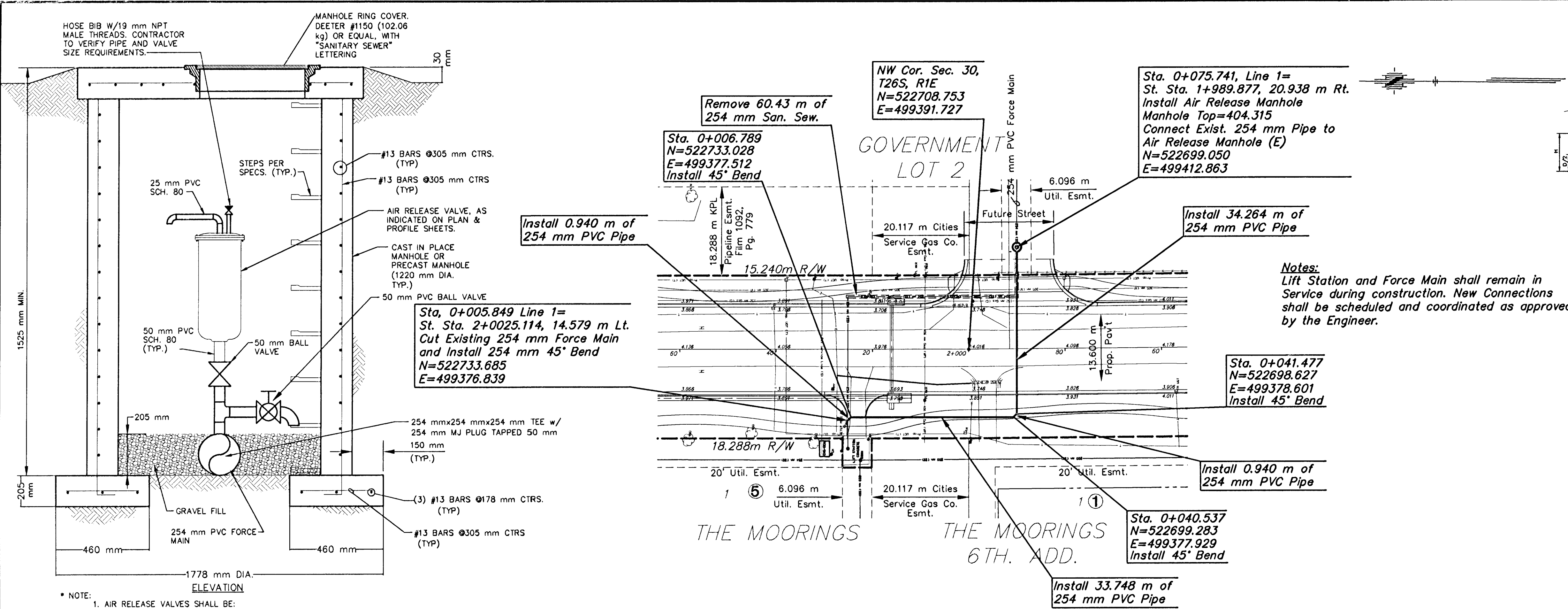
PLAN - LINE 1 SCALE: 1 : 500
