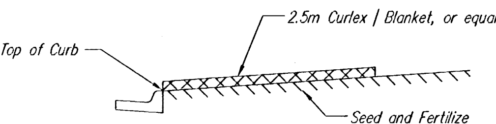
SECTION A-A
