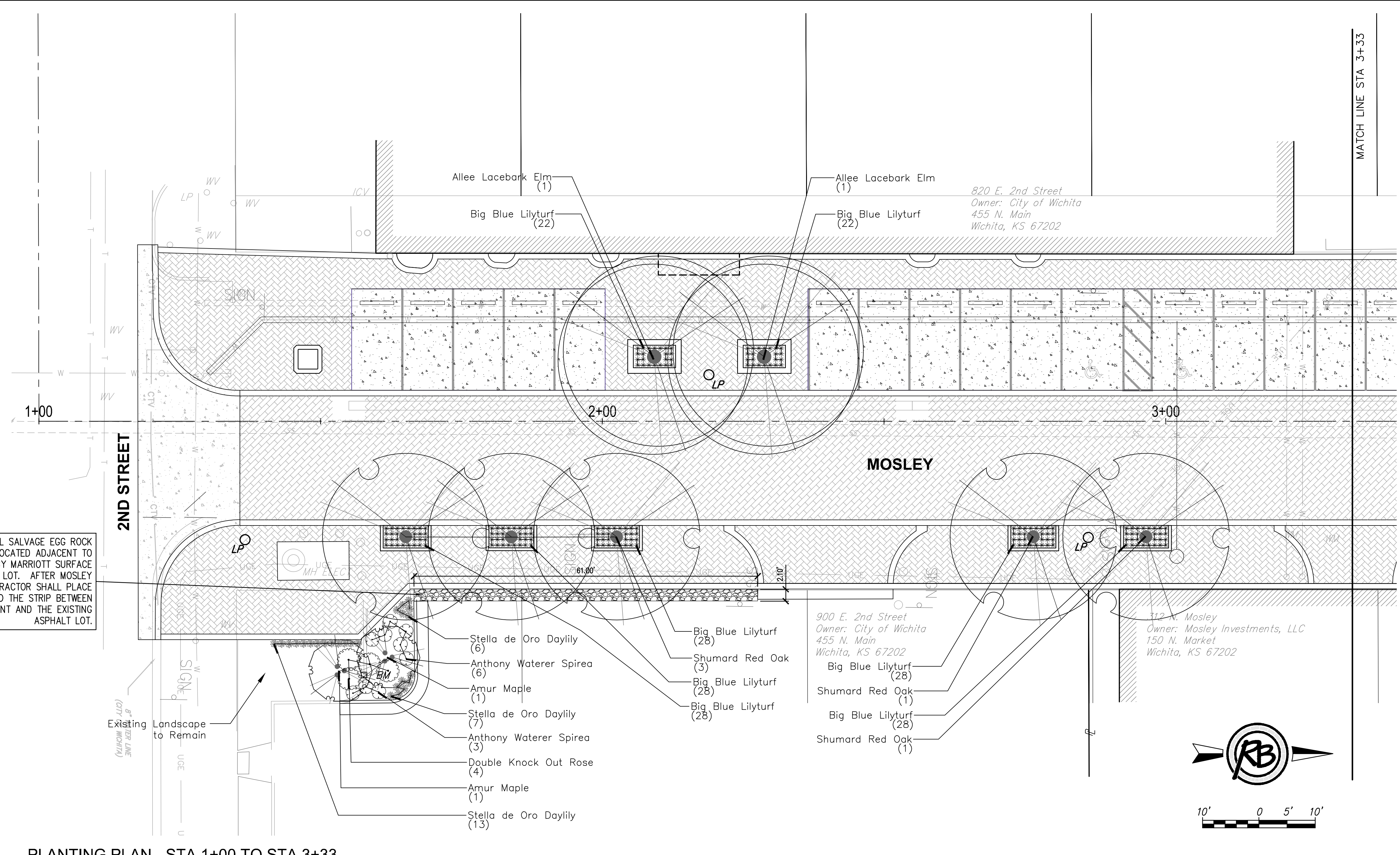
PLANTING PLAN - STA 1+00 TO STA 3+33 SCALE: 1" = 10'
