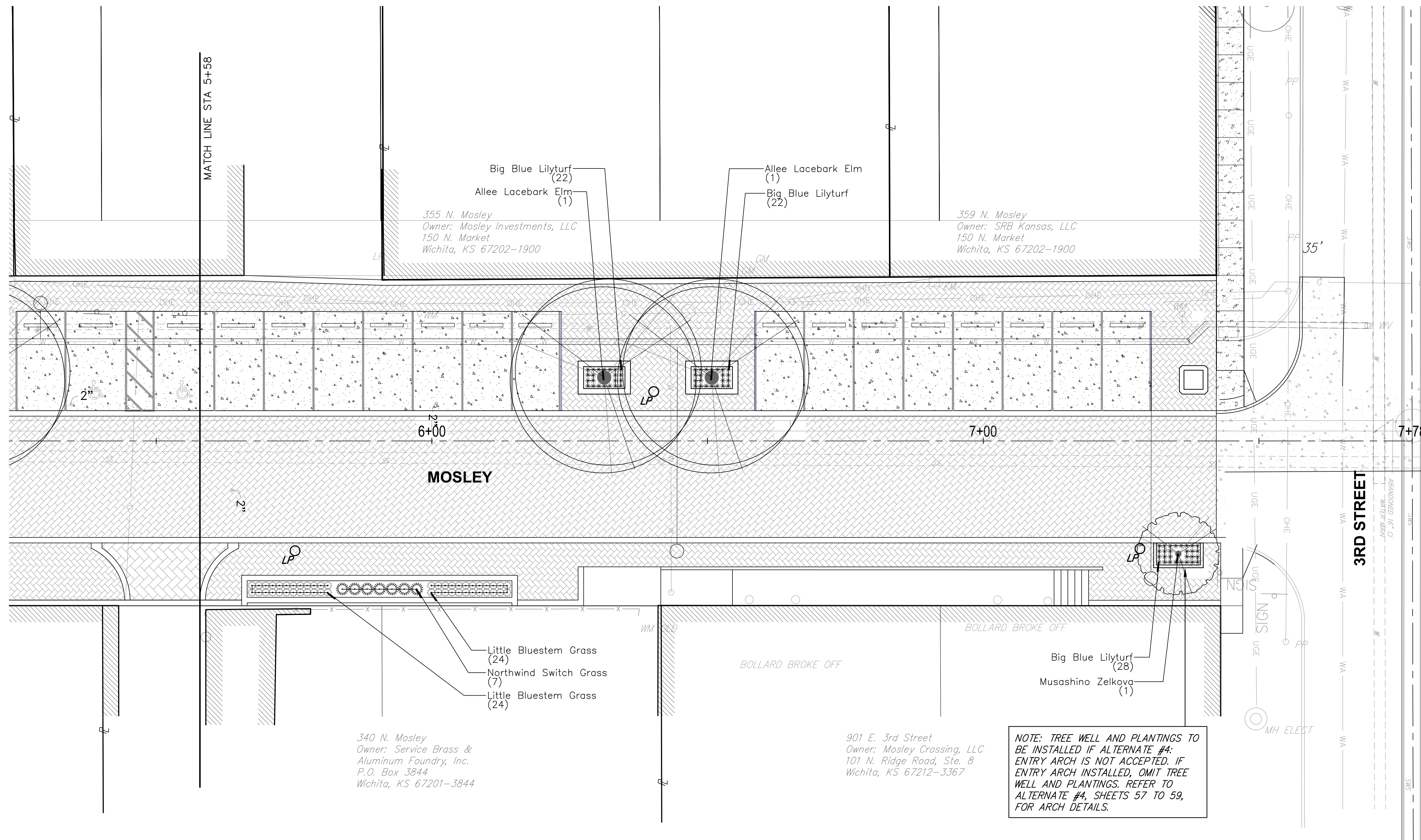
PLANTING PLAN - STA 5+58 TO STA 7+78 SCALE: 1" = 10'
