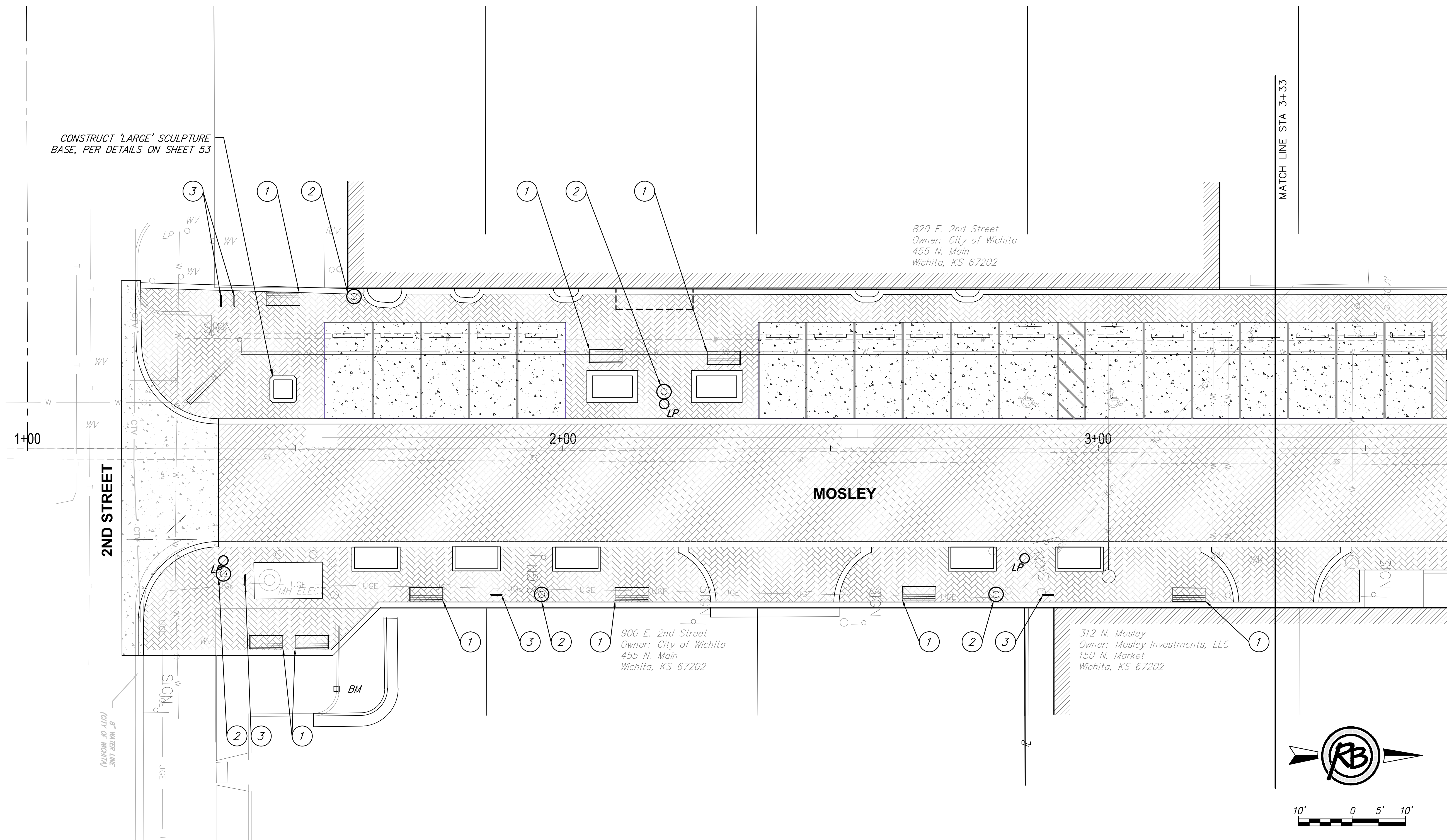
FURNISHINGS PLAN - STA 1+00 TO STA 3+33 SCALE: 1" = 10'
