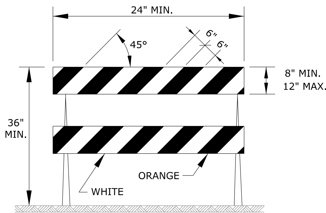
TYPE 2 BARRICADE
