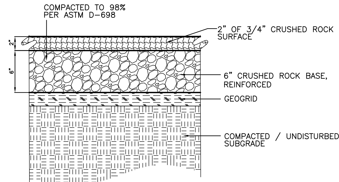
10 GRAVEL SECTION SCALE: NTS
