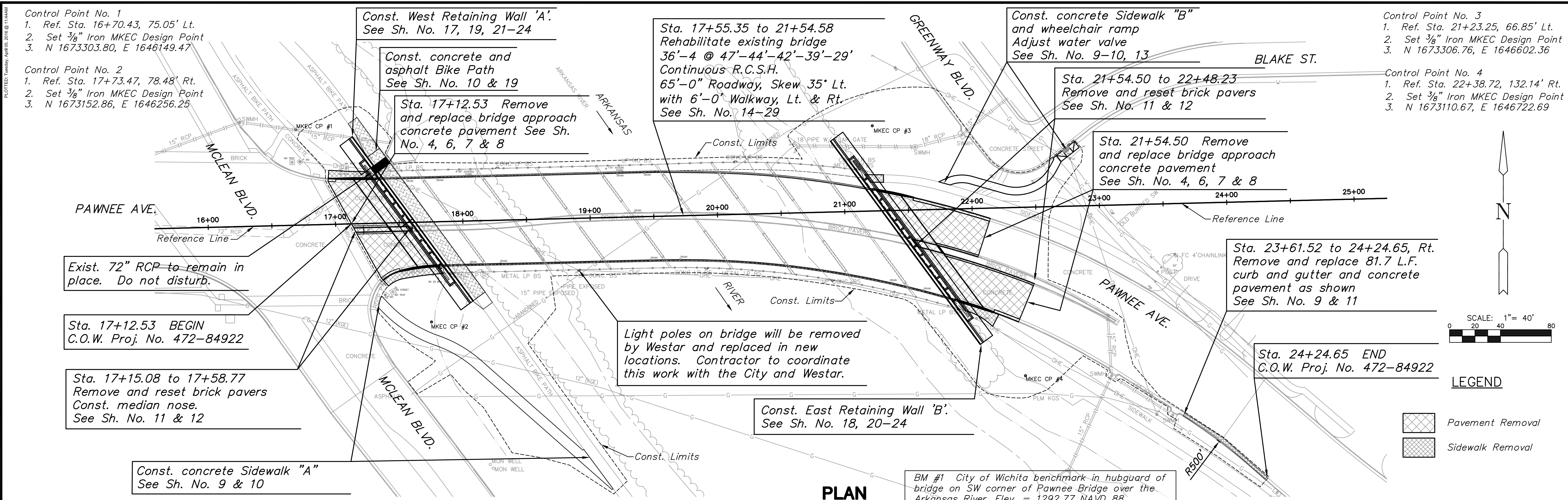
PLAN PROFILE SCALE: HORIZ. 1"=40' SCALE: VERT. 1"=5'
