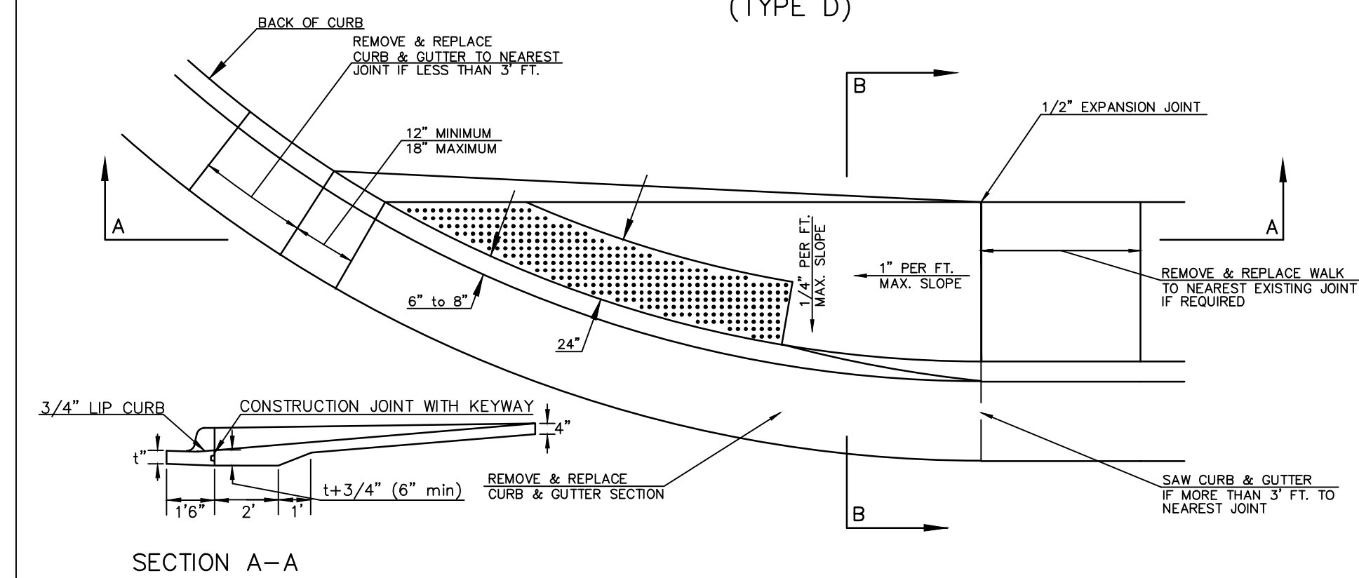
SECTION A-A
