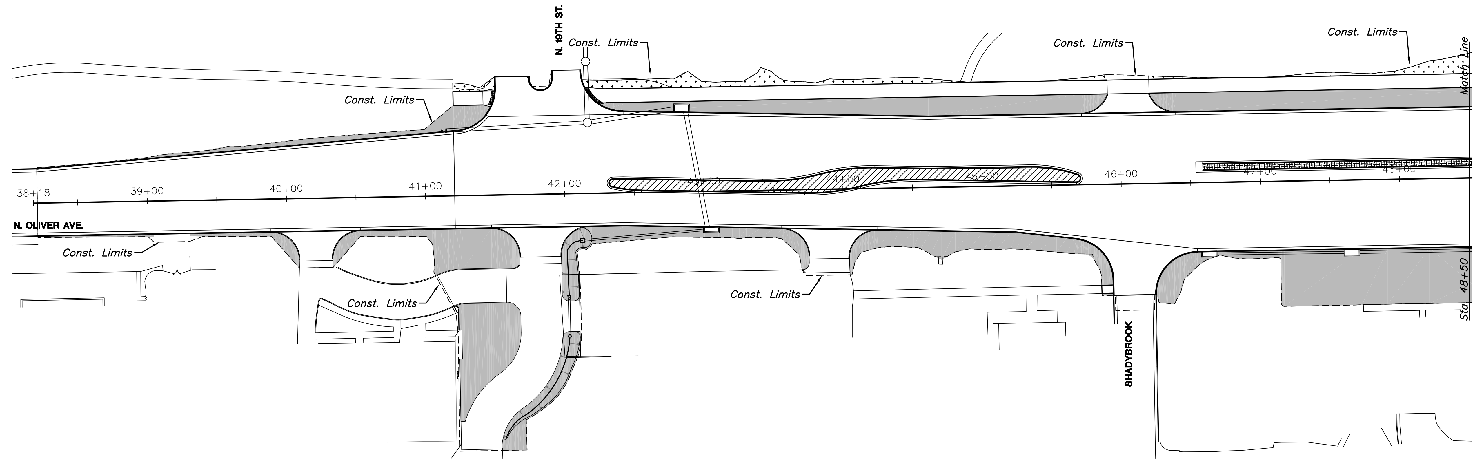
PLAN - N. OLIVER AVE.
