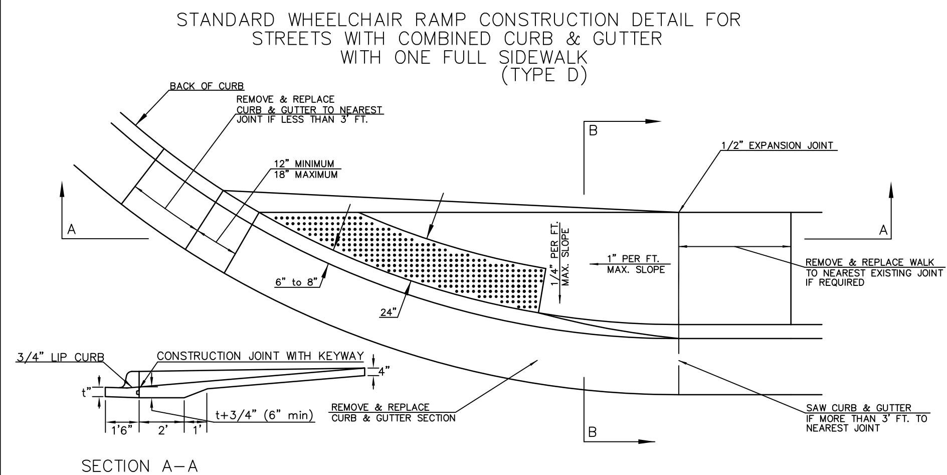
SECTION A-A
