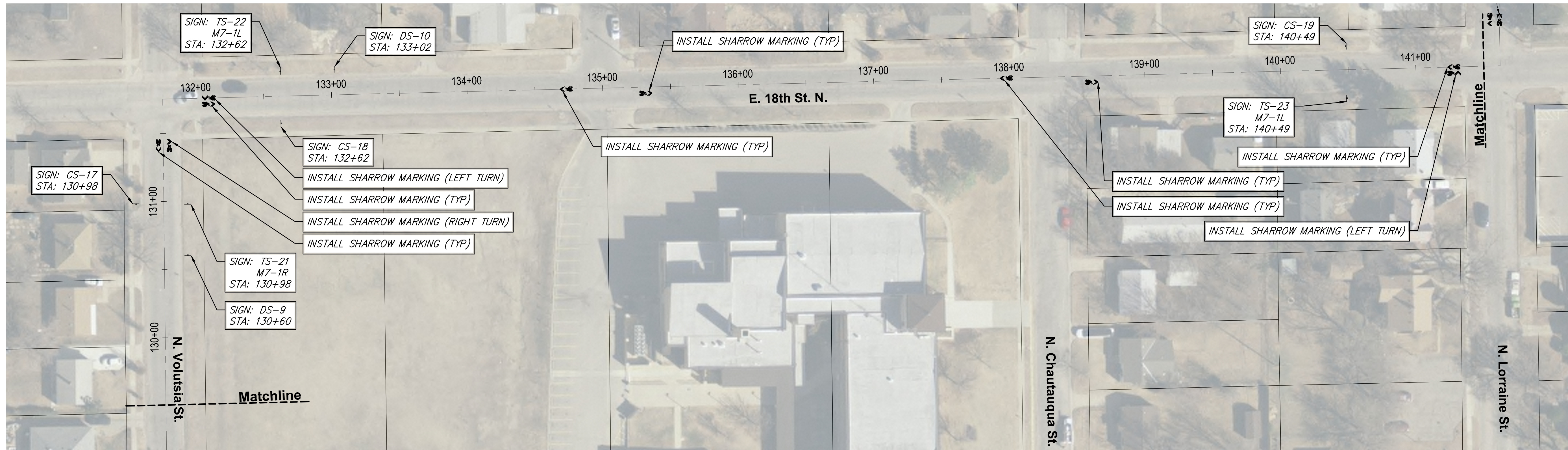
STA 129+50 TO STA 141+50 SCALE 1" = 40' - 0"
