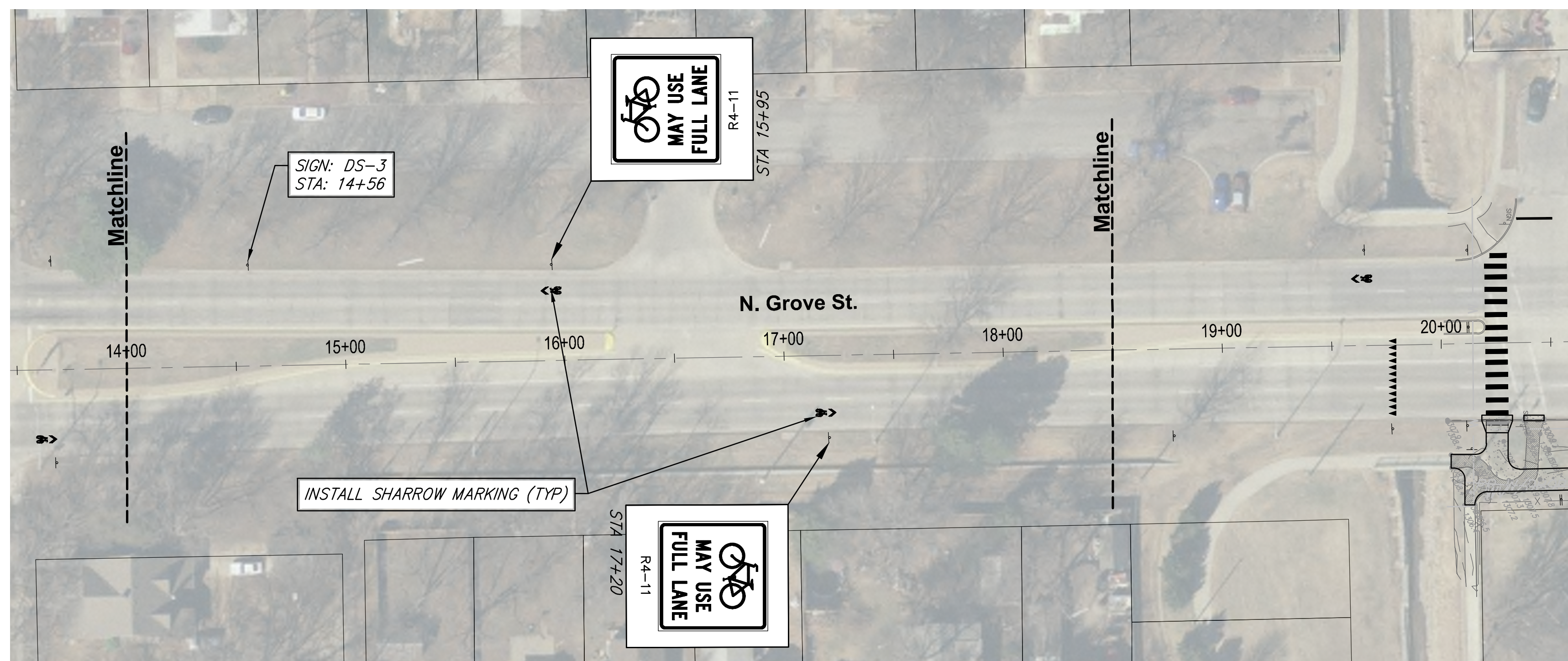
STA 14+00 TO STA 18+50 SCALE 1" = 40' - 0"
