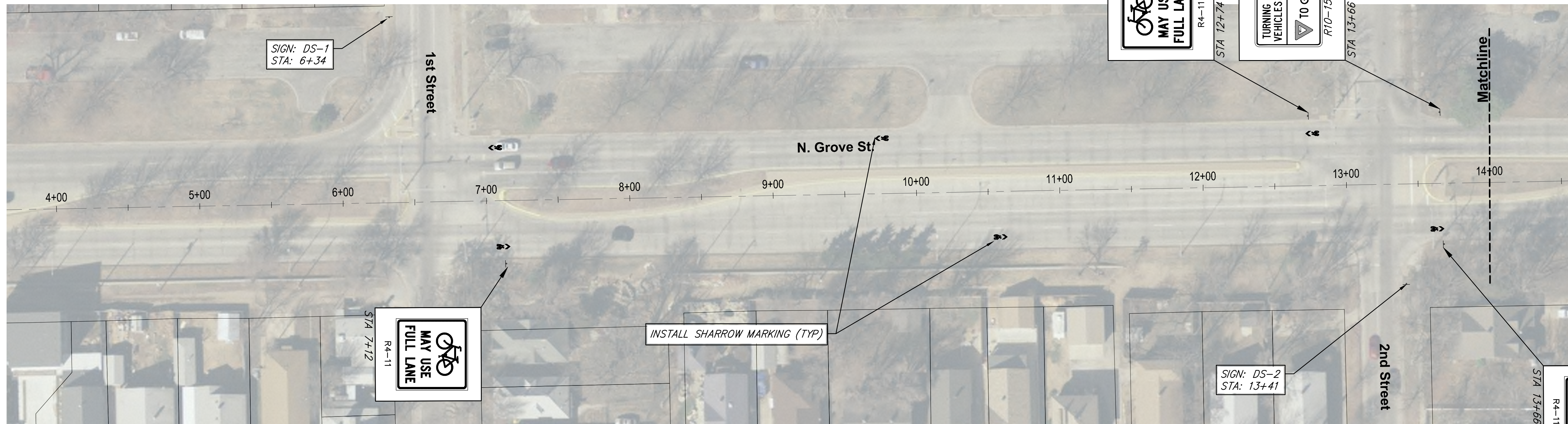
STA 5+00 TO STA 14+00 SCALE 1" = 40' - 0"
