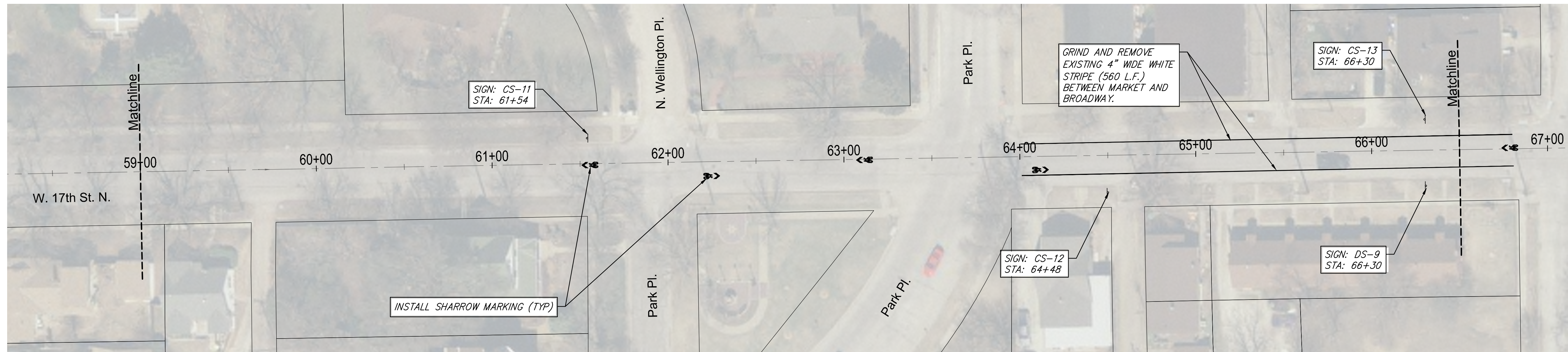
STA 59+00 TO STA 66+50
